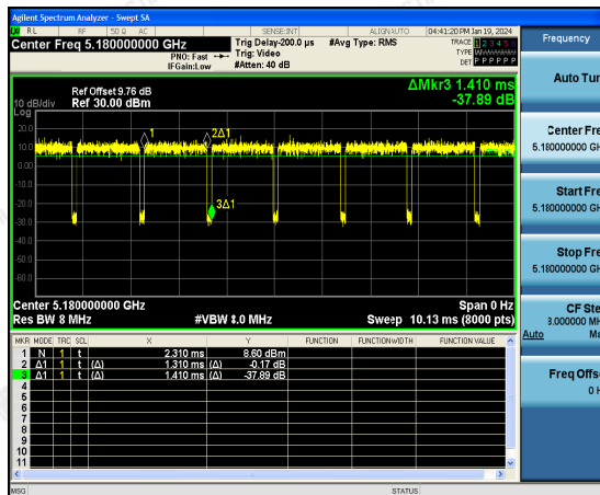
802.11ac(HT20)
