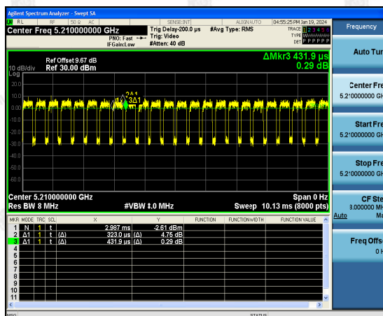
802.11ac(HT80)
