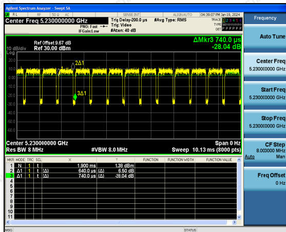
802.11n(HT40)
