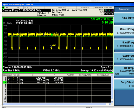
802.11ac(HT40)
