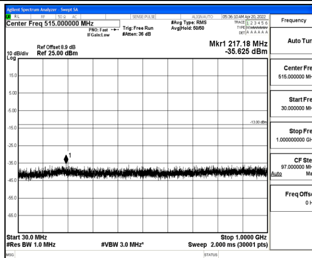
Band25-5MHz-QPSK-26365-1-0-Low-30-1000--35.63-PASS
