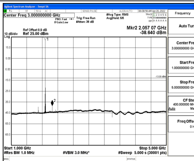
Band25-10MHz-QPSK-26365-1-0-Low-1000-5000--38.64-PASS
