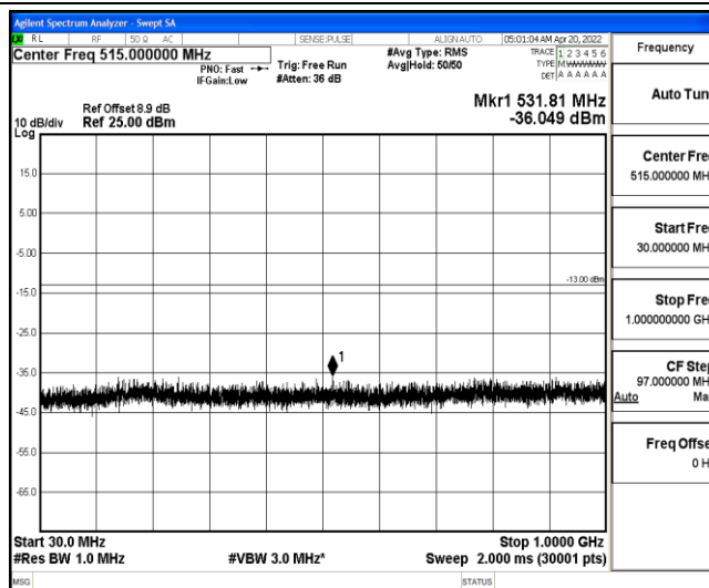
Band25-3MHz-16QAM-26055-1-0-Low-30-1000--36.05-PASS
