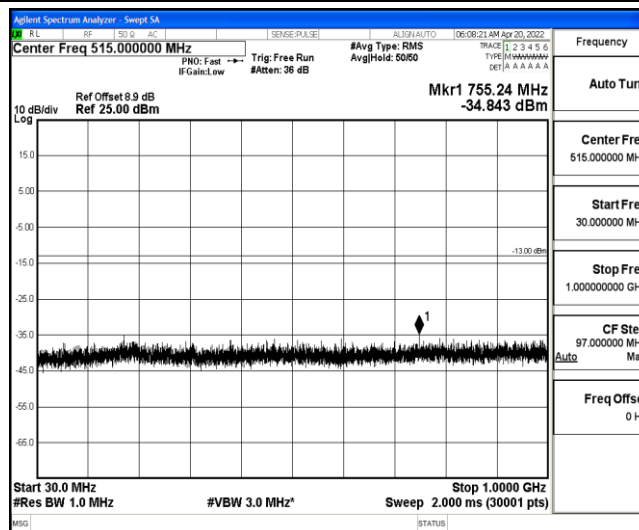
Band25-10MHz-QPSK-26365-1-0-Low-30-1000--34.84-PASS
