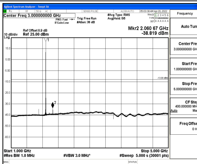
Band25-3MHz-QPSK-26365-1-0-Low-1000-5000--38.82-PASS
