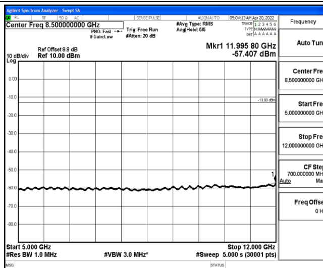
Band25-3MHz-QPSK-26365-1-0-Low-5000-12000--57.41-PASS
