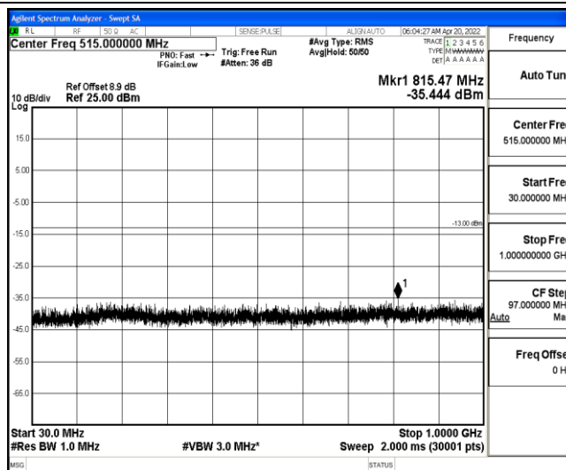
Band25-10MHz-QPSK-26090-1-0-Low-30-1000--35.44-PASS
