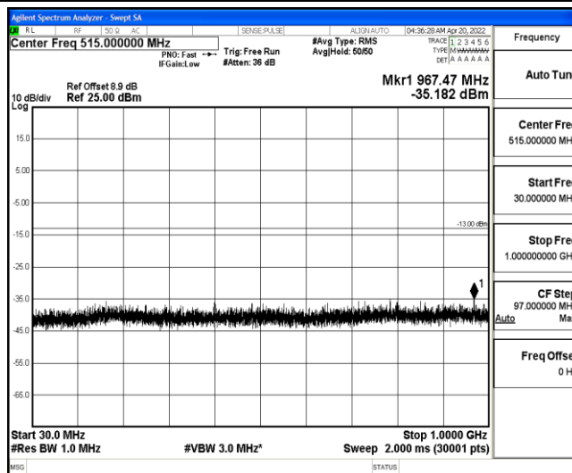
Band25-1.4MHz-QPSK-26365-1-0-Low-30-1000--35.18-PASS
