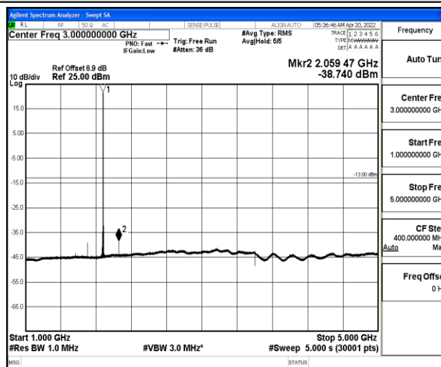
Band25-5MHz-QPSK-26365-1-0-Low-1000-5000--38.74-PASS
