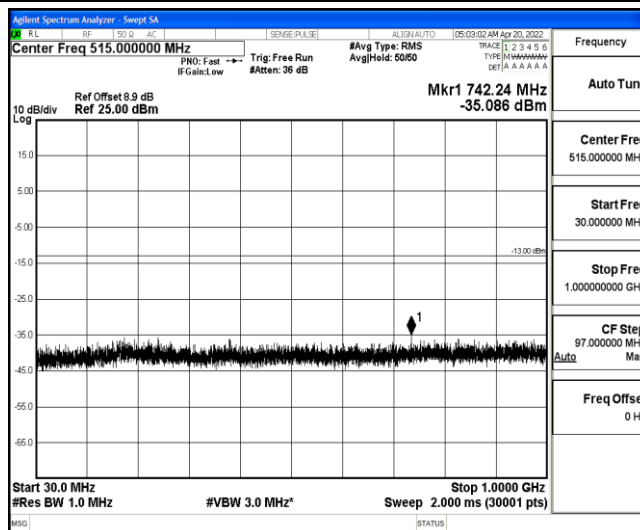
Band25-3MHz-QPSK-26365-1-0-Low-30-1000--35.09-PASS
