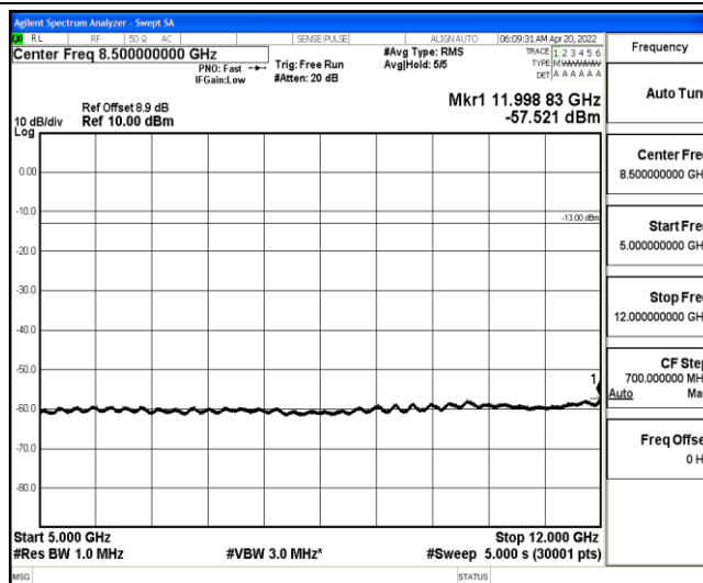
Band25-10MHz-QPSK-26365-1-0-Low-5000-12000--57.52-PASS
