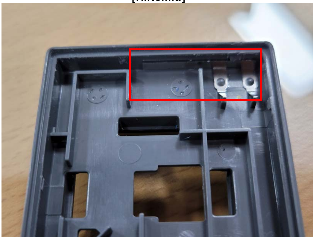
[Antenna]
