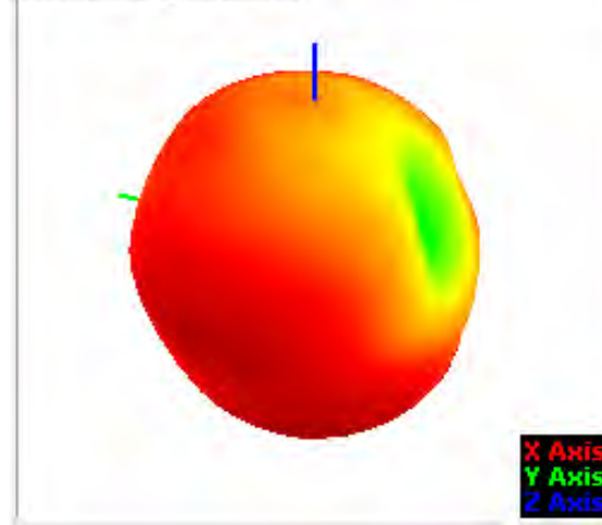
820.00MHz@T45P200
