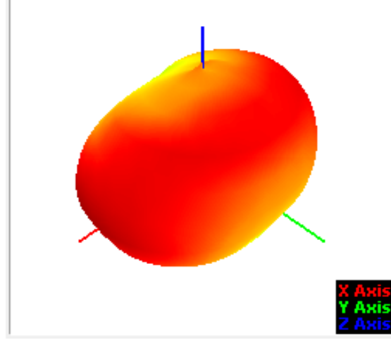
850.00MHz@T45P45
