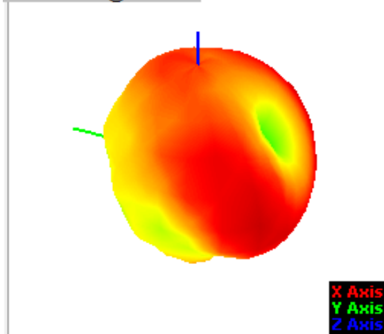
2300.00MHz@T45P200
