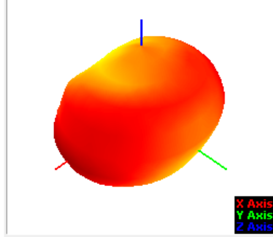
820.00MHz@T45P45
