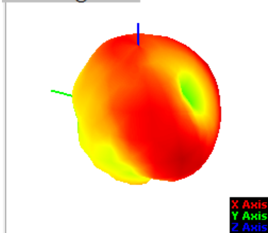
2320.00MHz@T45P200
