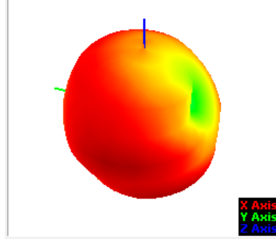
850.00MHz@T45P200
