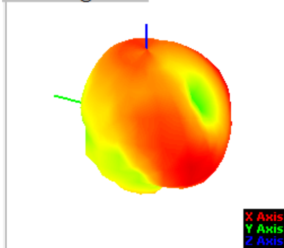
2340.00MHz@T45P200
