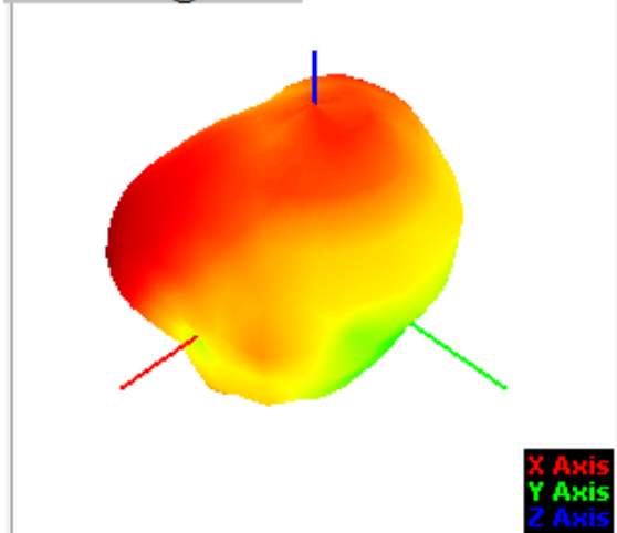
2300.00MHz@T45P45
