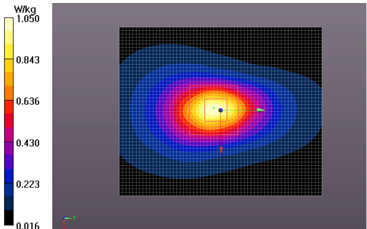
Fig.8 WCDMA1900 CH9538
