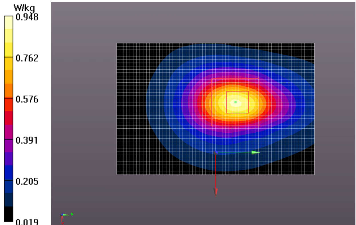
Fig.10 WCDMA1700
