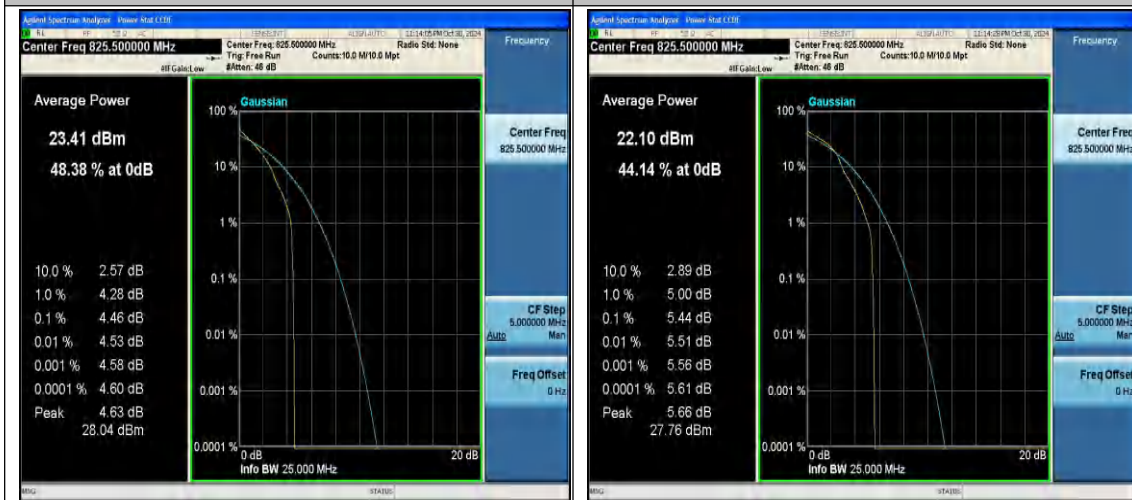
26(824-849)-3MHz-QPSK-26805-1RB#0-PASS
