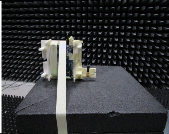
EUT Horizontal
