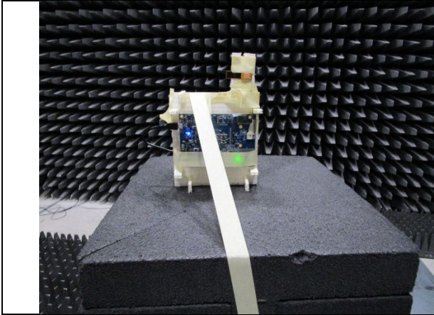
EUT Vertical
