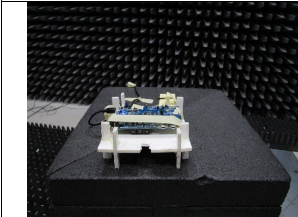
EUT Flat
