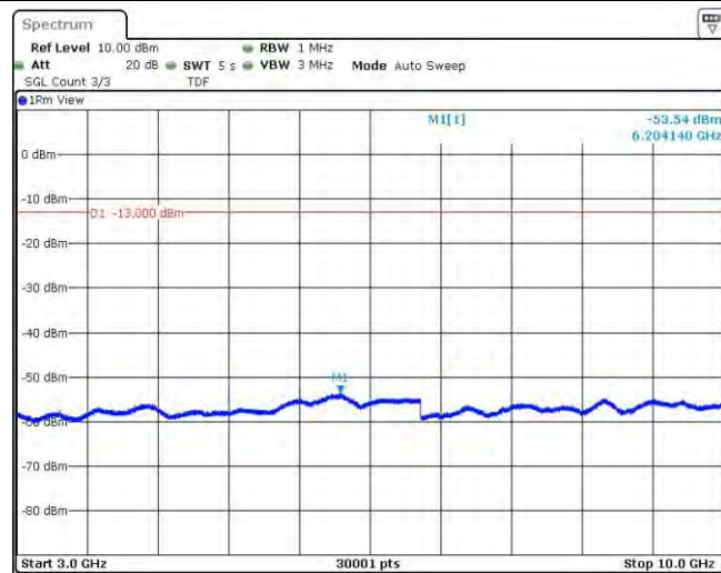
Band4-1312-4-3000~10000MHz
