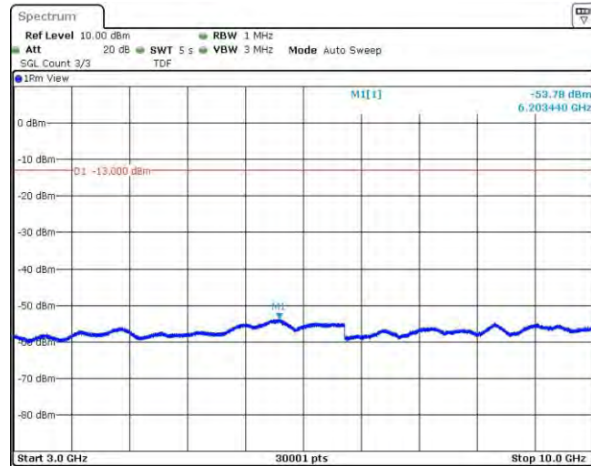
Band4-1413-1-1000~3000MHz
