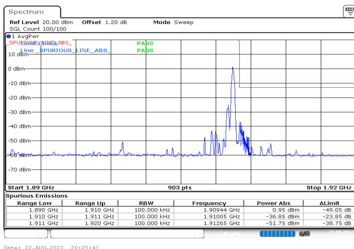
n2_20MHz_15kHz_1900MHz_DFT-s-OFDM QPSK_RB1@105
