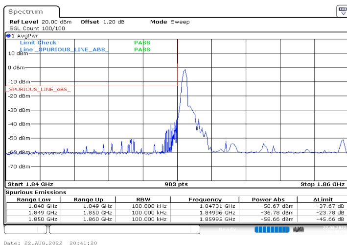
n2_10MHz_15kHz_1855MHz_DFT-s-OFDM QPSK_RB1@0
