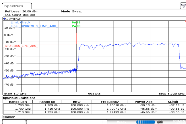
DC_12A_n66A_10MHz|15MHz_15kHz_707.5MHz|1717.5MHz_ DFT-s-OFDM QPSK_RB0|RB75@0
