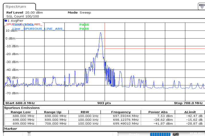
DC_2A_n71A_10MHz|10MHz_15kHz_1880MHz|693MHz_DF T-s-OFDM QPSK_RB0|RB1@51
