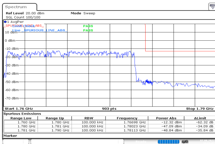
DC_12A_n66A_10MHz|20MHz_15kHz_707.5MHz|1770MHz_ DFT-s-OFDM QPSK_RB0|RB100@0
