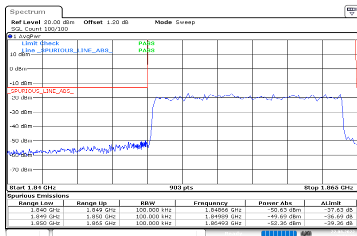
n2_15MHz_15kHz_1857.5MHz_DFT-s-OFDM QPSK_RB75@0
