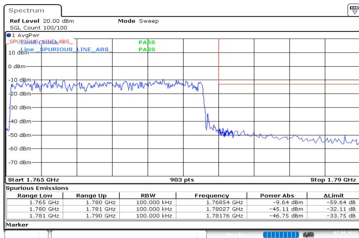
DC_12A_n66A_10MHz|15MHz_15kHz_707.5MHz|1772.5MHz_ DFT-s-OFDM QPSK_RB0|RB75@0
