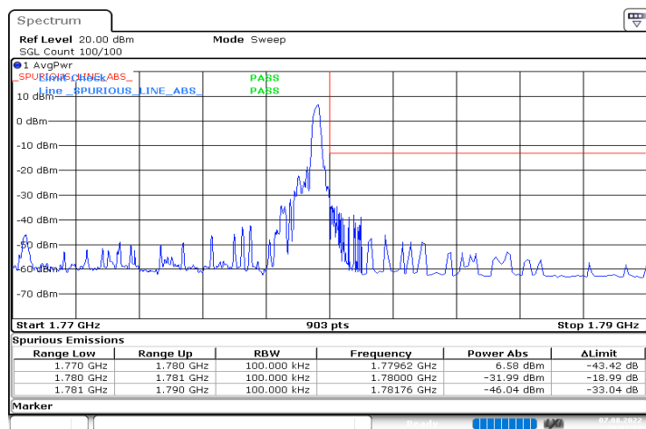
DC_12A_n66A_10MHz|10MHz_15kHz_707.5MHz|1775MHz_ DFT-s-OFDM QPSK_RB0|RB1@51
