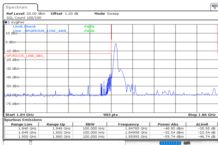
n2_10MHz_15kHz_1855MHz_DFT-s-OFDM QPSK_RB1@0
