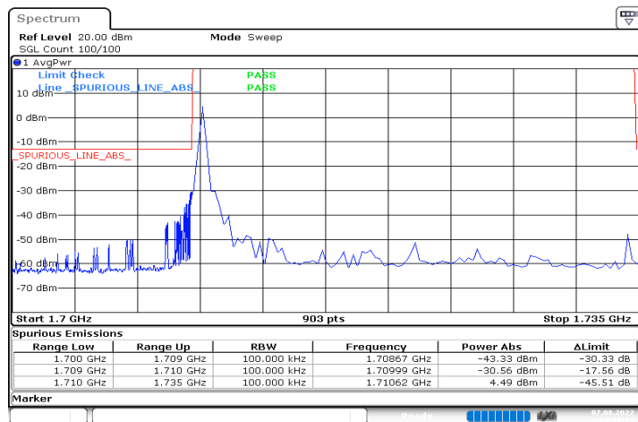
DC_12A_n66A_10MHz|25MHz_15kHz_707.5MHz|1722.5MHz_ _DFT-s-OFDM QPSK_RB0|RB1@0
