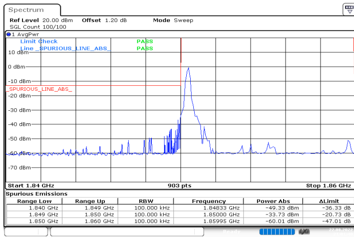
n2_10MHz_15kHz_1855MHz_DFT-s-OFDM QPSK_RB1@0
