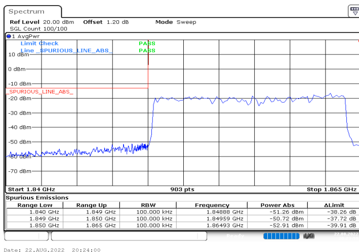
n2_15MHz_15kHz_1857.5MHz_DFT-s-OFDM QPSK_RB75@0
