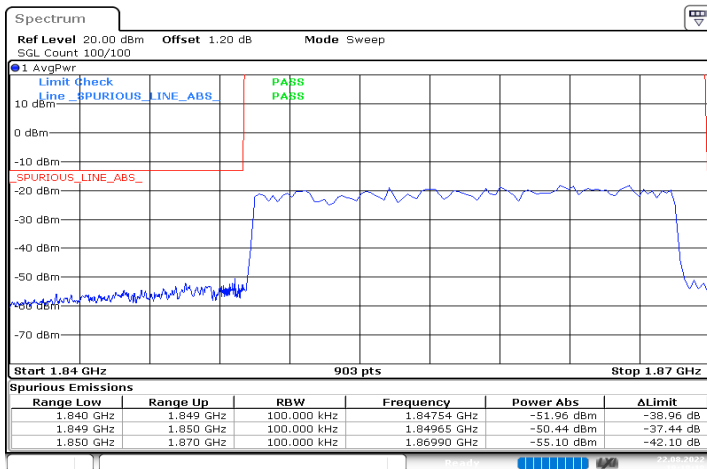
n25_20MHz_15kHz_1860MHz_DFT-s-OFDM QPSK_RB100@0
