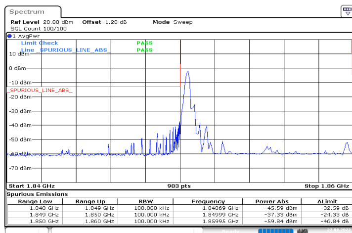
n2_10MHz_15kHz_1855MHz_DFT-s-OFDM QPSK_RB1@0
