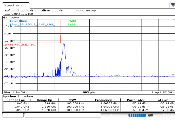
n25_20MHz_15kHz_1860MHz_DFT-s-OFDM QPSK_RB1@0
