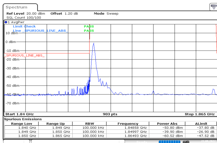
n2_15MHz_15kHz_1857.5MHz_DFT-s-OFDM QPSK_RB1@0
