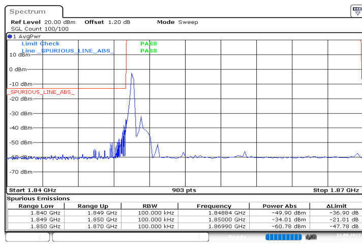
n2_20MHz_15kHz_1860MHz_DFT-s-OFDM QPSK_RB1@0
