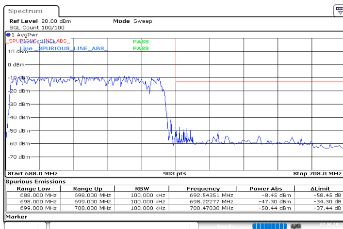
DC_2A_n71A_10MHz|10MHz_15kHz_1880MHz|693MHz_DF T-s-OFDM QPSK_RB0|RB50@0
