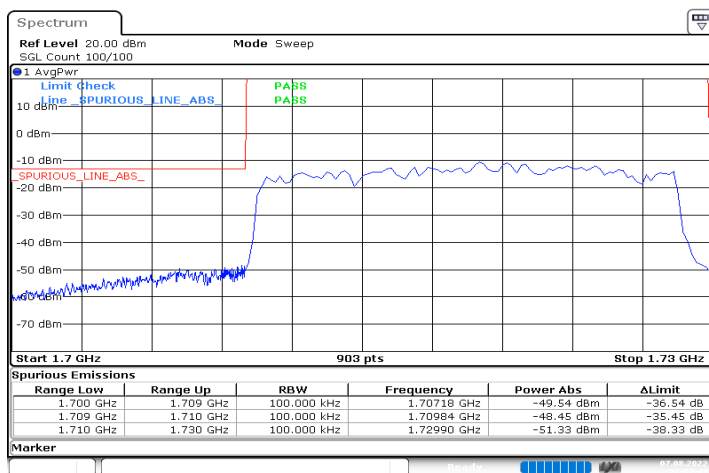
DC_12A_n66A_10MHz|20MHz_15kHz_707.5MHz|1720MHz_ DFT-s-OFDM QPSK_RB0|RB100@0
