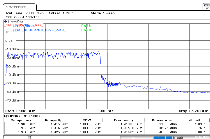
n25_10MHz_15kHz_1910MHz_DFT-s-OFDM QPSK_RB50@0
