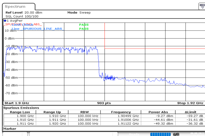
DC_12A_n2A_10MHz|10MHz_15kHz_707.5MHz|1905MHz_D FT-s-OFDM QPSK_RB0|RB50@0
