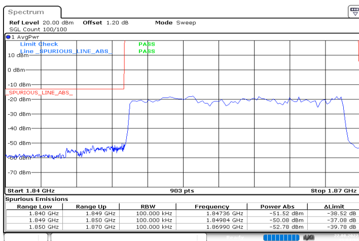
n2_20MHz_15kHz_1860MHz_DFT-s-OFDM QPSK_RB100@0
