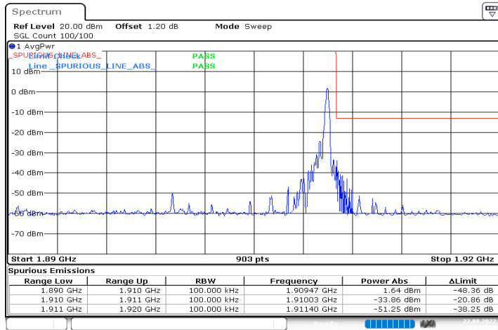
n2_20MHz_15kHz_1900MHz_DFT-s-OFDM QPSK_RB1@105
