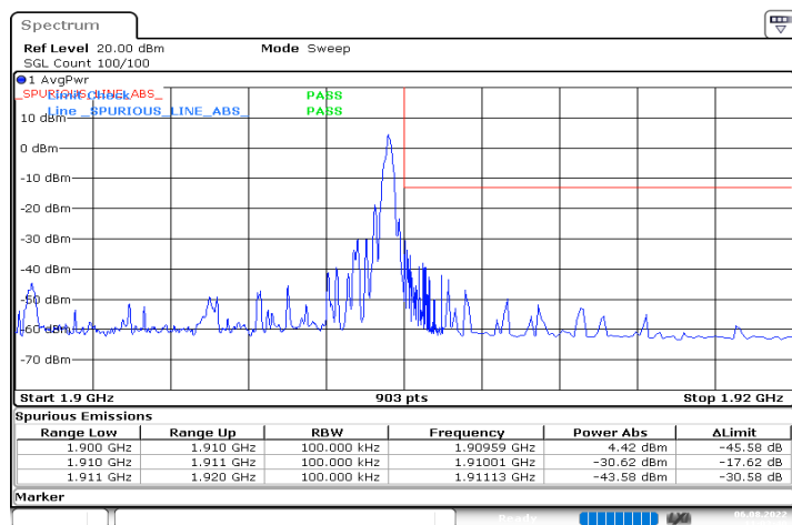
DC_12A_n2A_10MHz|10MHz_15kHz_707.5MHz|1905MHz_D FT-s-OFDM QPSK_RB0|RB1@51
