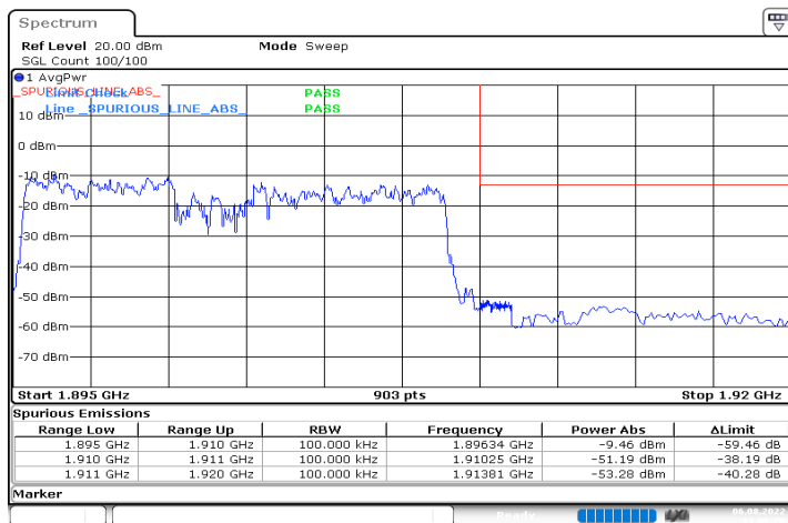
DC_12A_n2A_10MHz|15MHz_15kHz_707.5MHz|1902.5MHz_ DFT-s-OFDM QPSK_RB0|RB75@0
