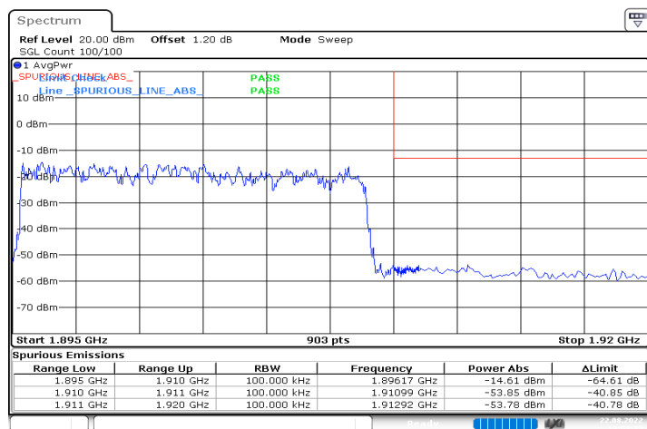
n2_15MHz_15kHz_1902.5MHz_DFT-s-OFDM QPSK_RB75@0
