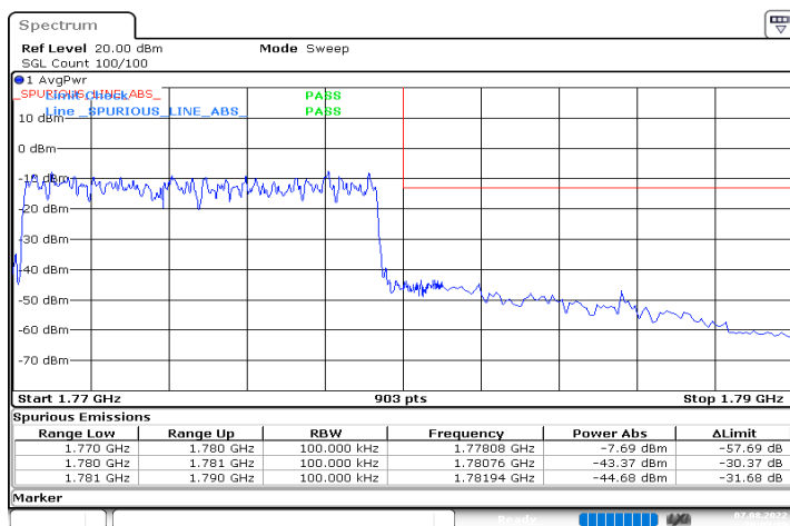
DC_12A_n66A_10MHz|10MHz_15kHz_707.5MHz|1775MHz_ DFT-s-OFDM QPSK_RB0|RB50@0
