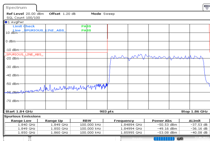
n2_10MHz_15kHz_1855MHz_DFT-s-OFDM QPSK_RB50@0
