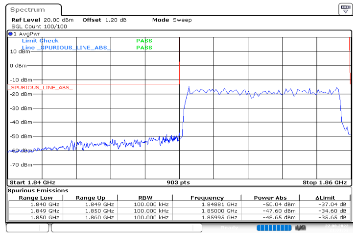
n2_10MHz_15kHz_1855MHz_DFT-s-OFDM QPSK_RB50@0
