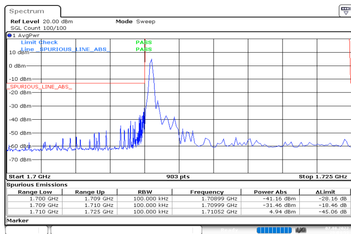
DC_12A_n66A_10MHz|15MHz_15kHz_707.5MHz|1717.5MHz_ DFT-s-OFDM QPSK_RB0|RB1@0
