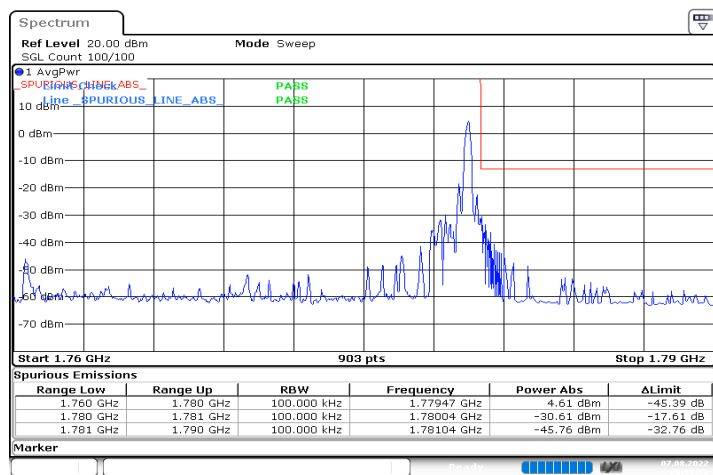
DC_12A_n66A_10MHz|20MHz_15kHz_707.5MHz|1770MHz_ DFT-s-OFDM QPSK_RB0|RB1@105
