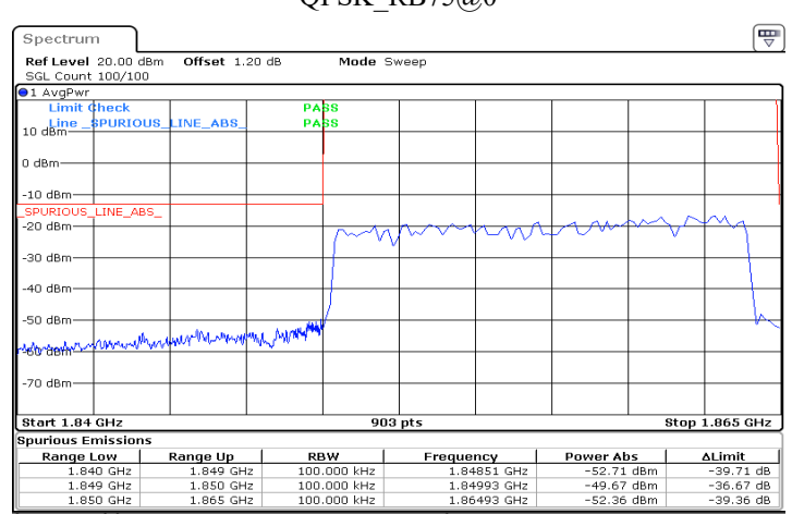
n2_15MHz_15kHz_1857.5MHz_DFT-s-OFDM QPSK_RB75@0
