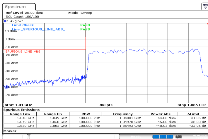
DC_12A_n2A_10MHz|15MHz_15kHz_707.5MHz|1857.5MHz_ DFT-s-OFDM QPSK_RB0|RB75@0
