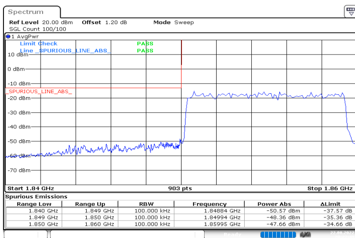
n2_10MHz_15kHz_1855MHz_DFT-s-OFDM QPSK_RB50@0
