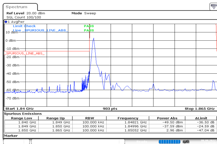
DC_12A_n2A_10MHz|15MHz_15kHz_707.5MHz|1857.5MHz_ DFT-s-OFDM QPSK_RB0|RB1@0
