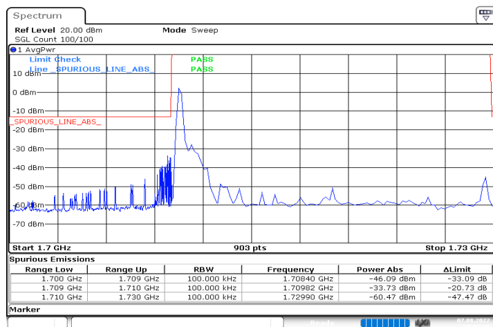
DC_12A_n66A_10MHz|20MHz_15kHz_707.5MHz|1720MHz_ DFT-s-OFDM QPSK_RB0|RB1@0
