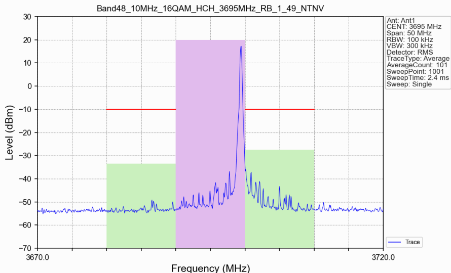
Band48_10MHz_16QAM_HCH_3695MHz_RB_1_49_NTNV
