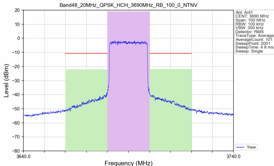
Band48_20MHz_QPSK_HCH_3690MHz_RB_100_0_NTNV
