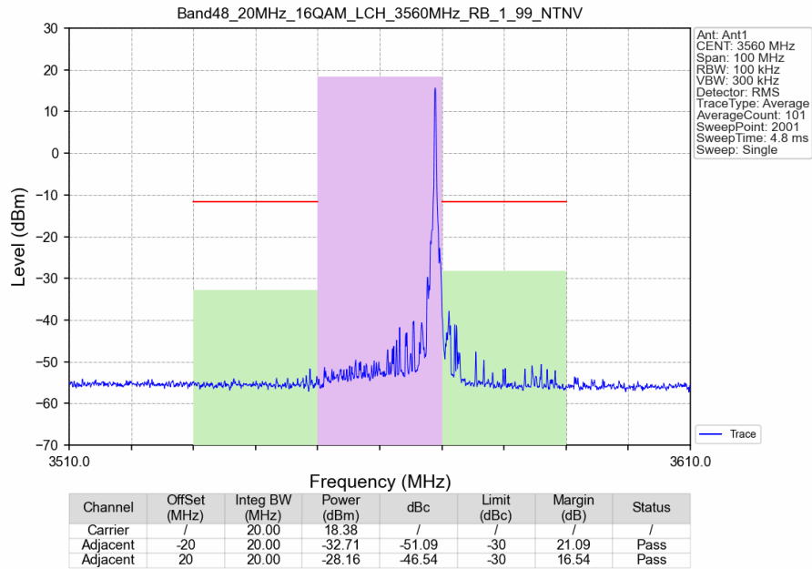
Band48_20MHz_16QAM_LCH_3560MHz_RB_1_99_NTNV
