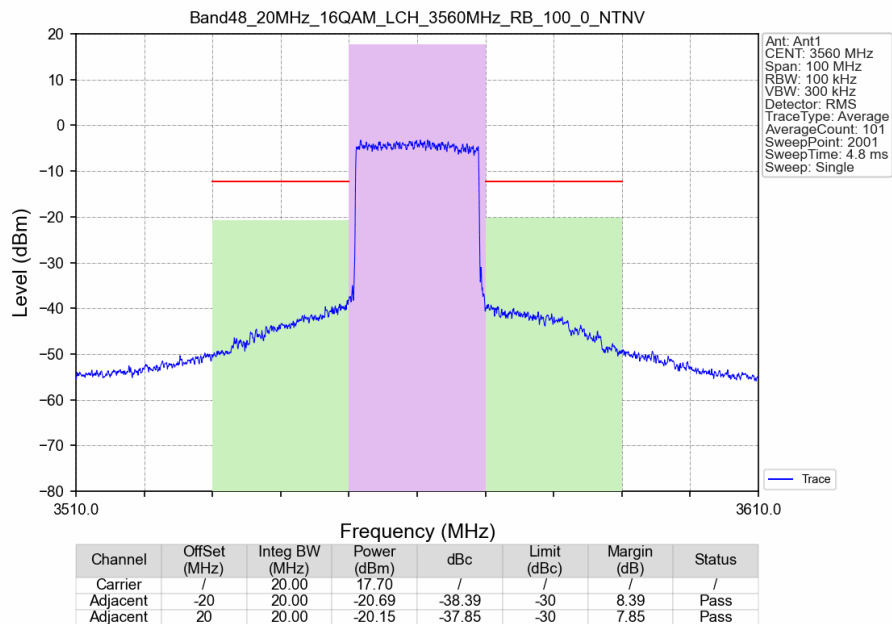
Band48_20MHz_16QAM_LCH_3560MHz_RB_100_0_NTNV
