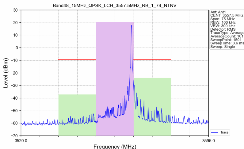
Band48_15MHz_QPSK_LCH_3557.5MHz_RB_1_74_NTNV
