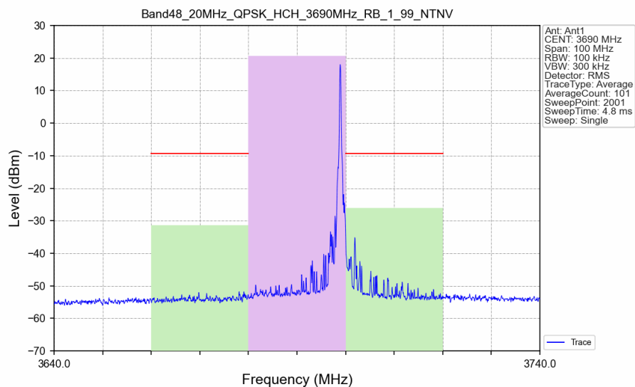
Band48_20MHz_QPSK_HCH_3690MHz_RB_1_99_NTNV
