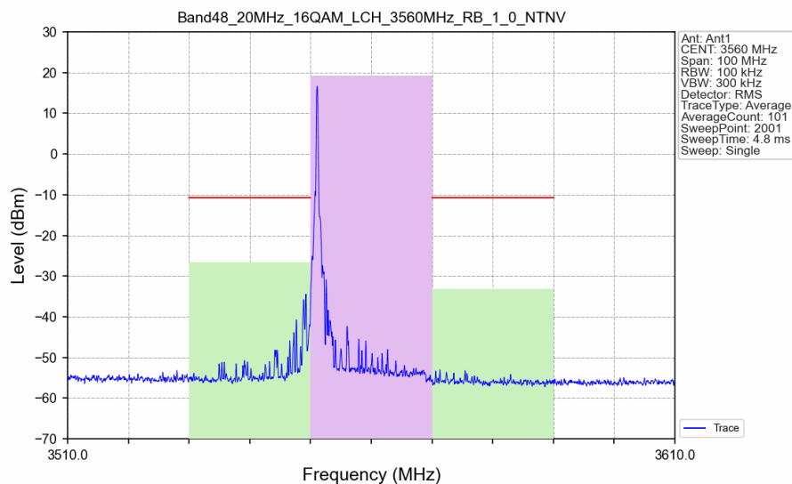
Band48_20MHz_16QAM_LCH_3560MHz_RB_1_0_NTNV
