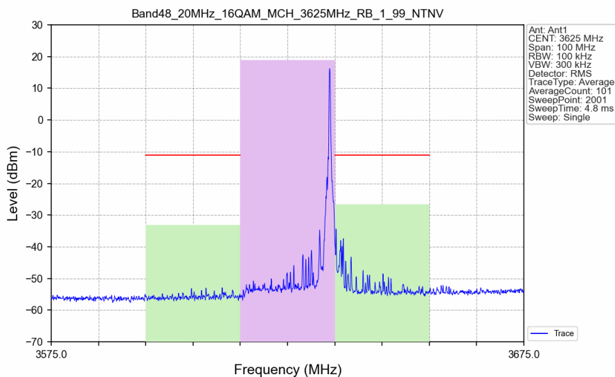
Band48_20MHz_16QAM_MCH_3625MHz_RB_1_99_NTNV
