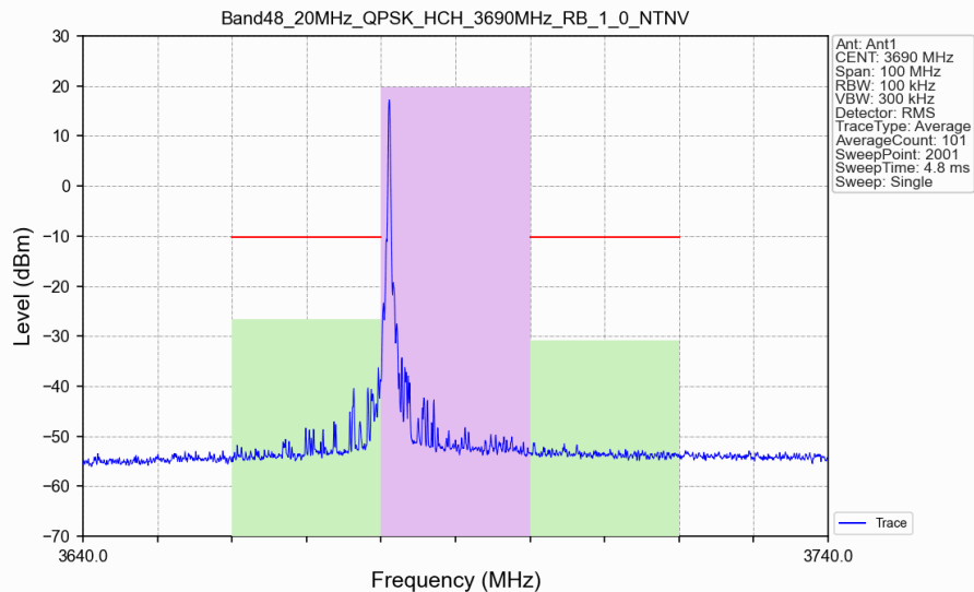
Band48_20MHz_QPSK_HCH_3690MHz_RB_1_0_NTNV
