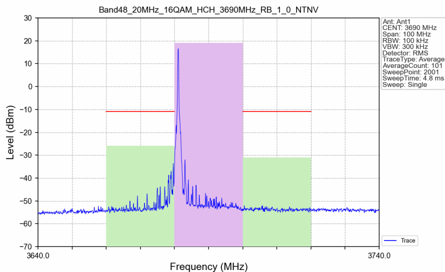
Band48_20MHz_16QAM_HCH_3690MHz_RB_1_0_NTNV
