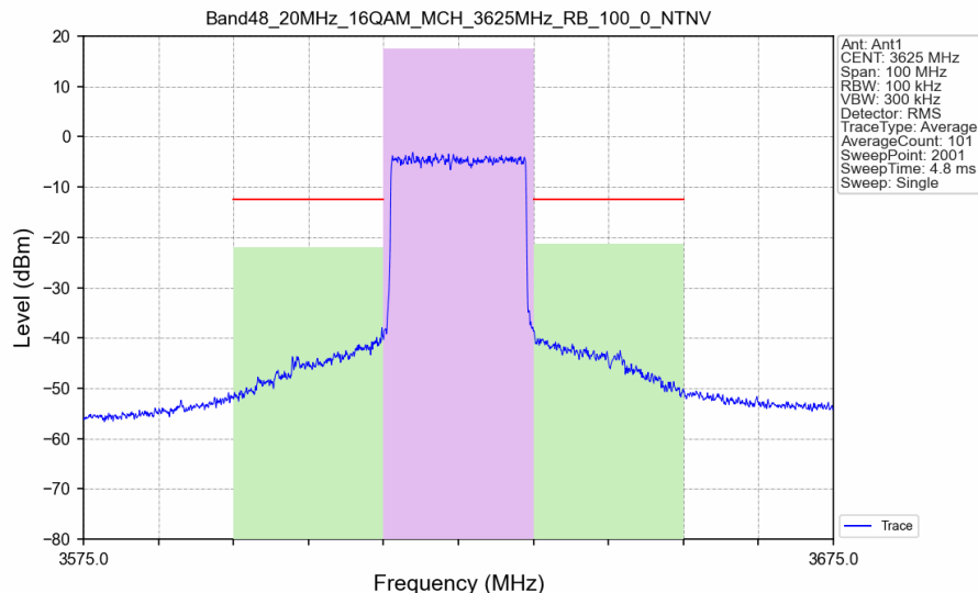
Band48_20MHz_16QAM_MCH_3625MHz_RB_100_0_NTNV
