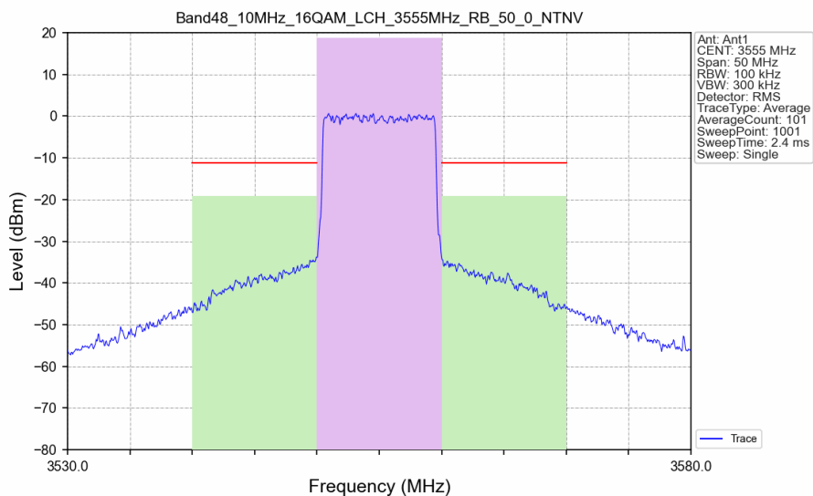
Band48_10MHz_16QAM_LCH_3555MHz_RB_50_0_NTNV
