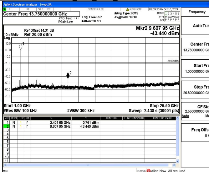
DH5_Ant1_2402_1000~26500
