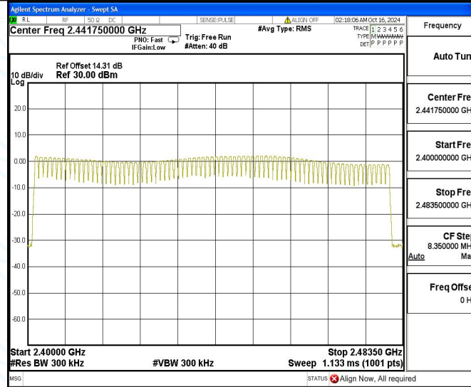
2DH5_Ant1_Hop
