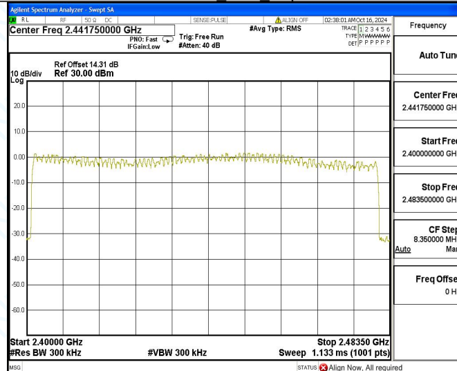
3DH5_Ant1_Hop
