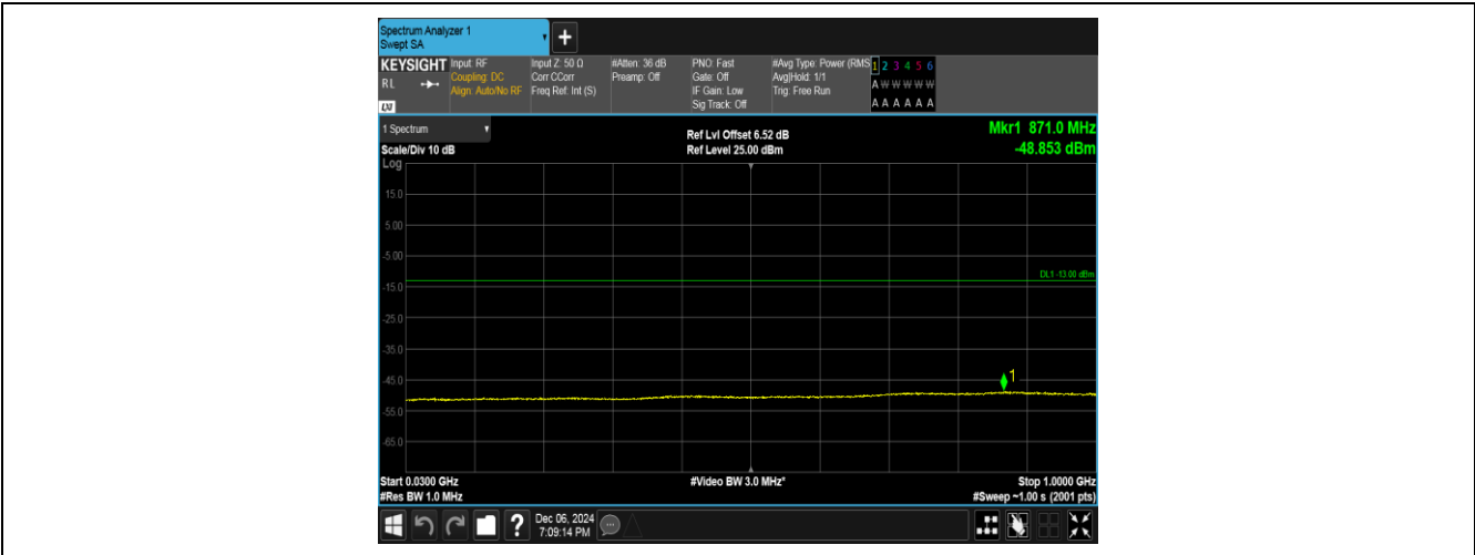
Band4-1413-4-30~1000MHz-PASS
