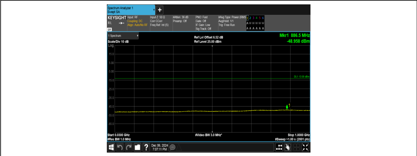
Band4-1413-3-30~1000MHz-PASS
