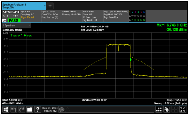
Figure 317 - A (Core 0) 802.11ax HE160 SU VLP 6665 MHz (CH143)
