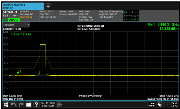
Figure 339 - A (Core 0) 802.11ax HE40 SU LPI 6165 MHz (CH43)
