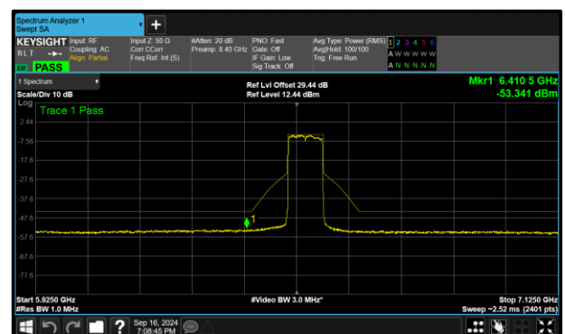
Figure 300 - A (Core 0) 802.11ax HE80 SU LPI 6545 MHz (CH119)
