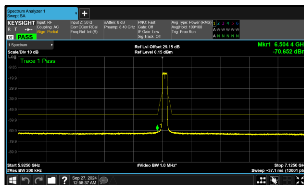
Figure 314 - A (Core 0) 802.11ax HE20 SU VLP 6535 MHz (CH117)
