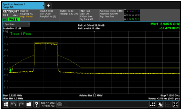
Figure 341 - A (Core 0) 802.11ax HE160 SU LPI 6185 MHz (CH47)
