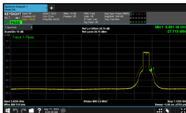
Figure 328 - A (Core 0) 802.11ax HE40 SU SP 6845 MHz (CH179)
