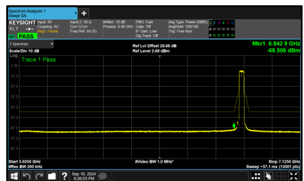
Figure 298 - A (Core 0) 802.11ax HE20 SU LPI 6875 MHz (CH185)
