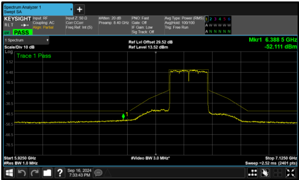
Figure 301 - A (Core 0) 802.11ax HE160 SU LPI 6665 MHz (CH143)
