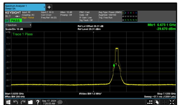
Figure 306 - A (Core 0) 802.11ax HE20 SU SP 6695 MHz (CH149)
