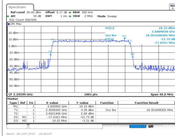
n41 SCS=30kHz CP_QAM256 BW=20MHz Channel=518598 RB=51@0
