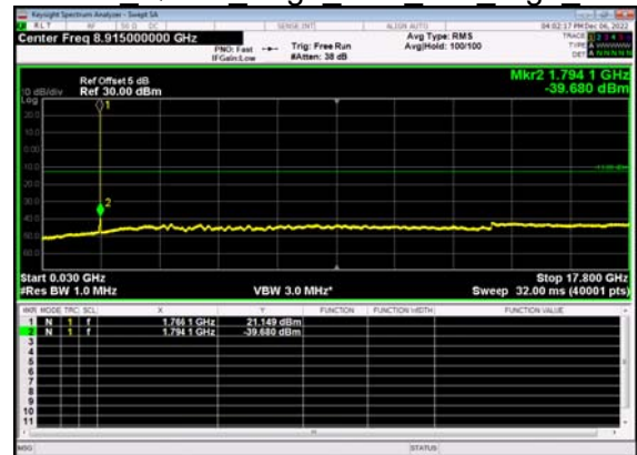
N66(15M)_DFT-s- OFDM QPSK Edge 1RB Left High CH
