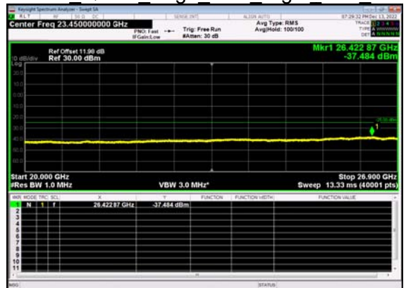
N41(100M)_DFT-s-OFDM QPSK Edge 1RB Right Low CH
