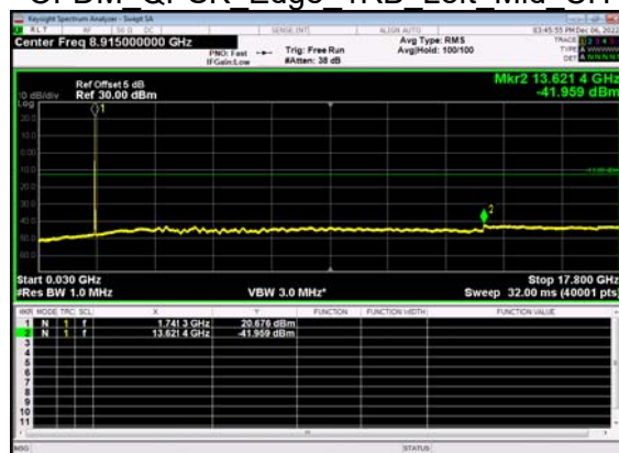
N66(10M)_DFT-s- OFDM QPSK Edge 1RB Left Mid CH
