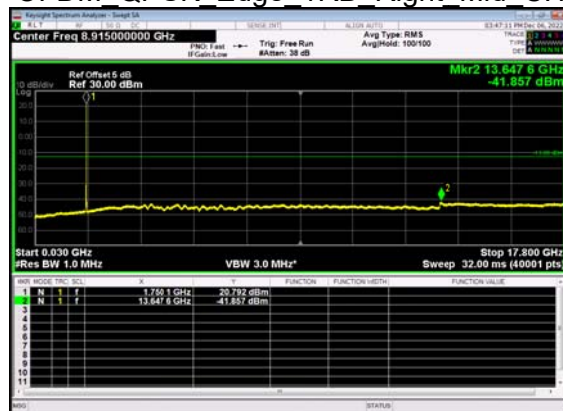
N66(10M)_DFT-s- OFDM QPSK Edge 1RB Right Mid CH
