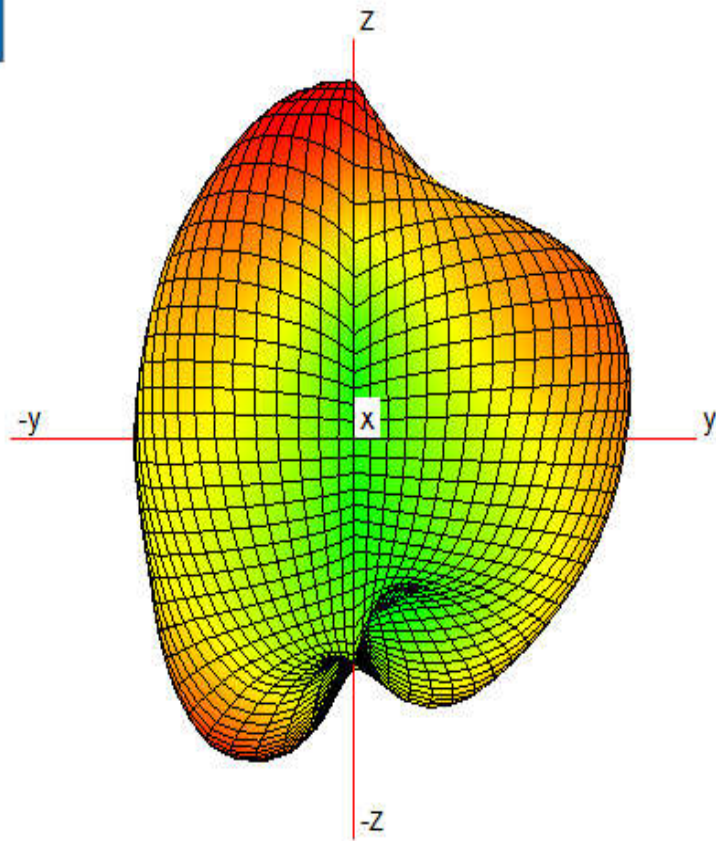
WIFI 5500MHz
