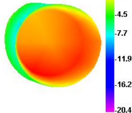
2450.000MHz E1
