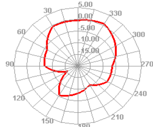
2450.000MHz E2
