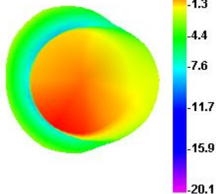
2400.000MHz E1
