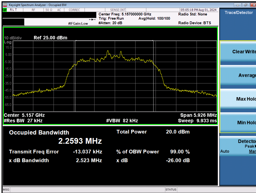
Plot 7-7. 26dB BW & 99% OBW (NB UNII HDR4 – 5157MHz)
