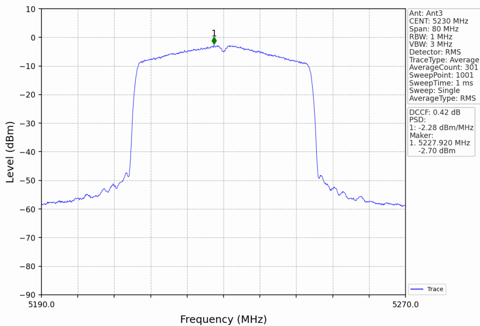
802.11ax(HEW40)_HCH_5230MHz_RU484_Left_Ant3_NTNV
