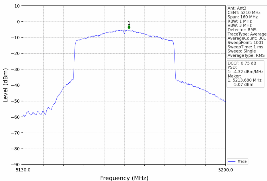
802.11ax(HEW80)_MCH_5210MHz_RU996_Left_Ant3_NTNV
