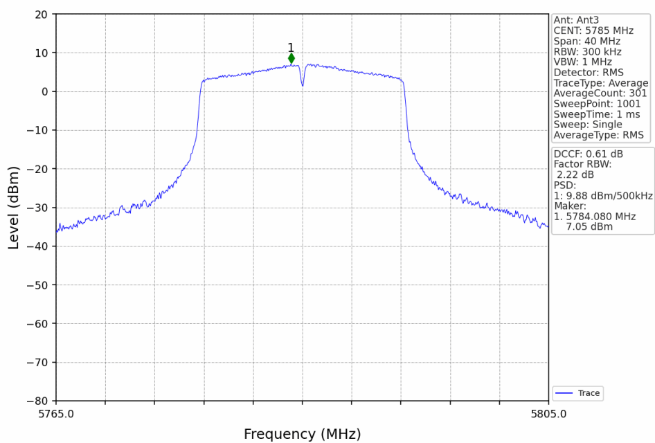
802.11a_MCH_5785MHz_Ant3_NTNV
