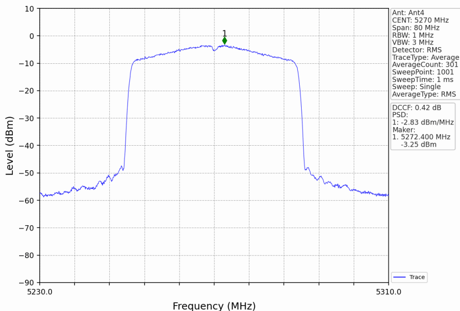
802.11ax(HEW40)_LCH_5270MHz_RU484_Left_Ant4_NTNV
