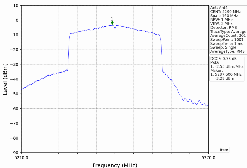
802.11ax(HEW80)_MCH_5290MHz_RU996_Left_Ant4_NTNV
