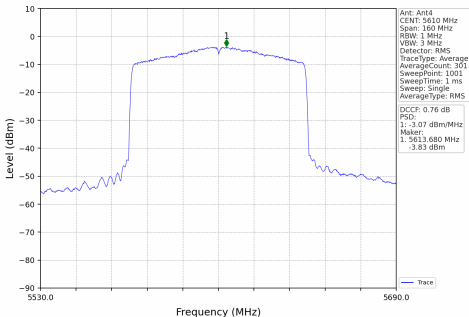
802.11ax(HEW80)_HCH_5610MHz_RU996_Left_Ant4_NTNV
