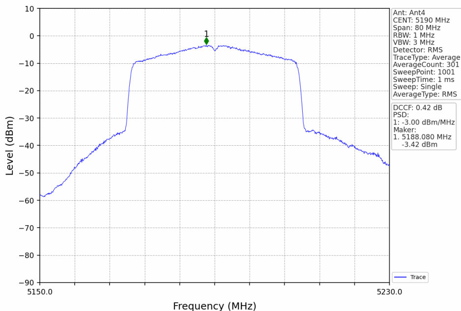
802.11ax(HEW40)_LCH_5190MHz_RU484_Left_Ant4_NTNV
