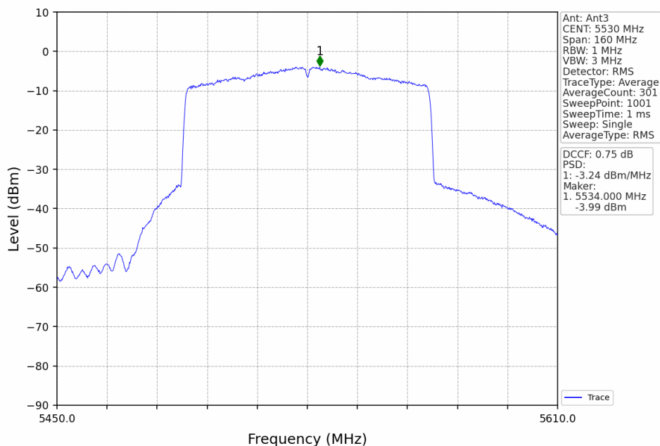
802.11ax(HEW80)_LCH_5530MHz_RU996_Left_Ant3_NTNV
