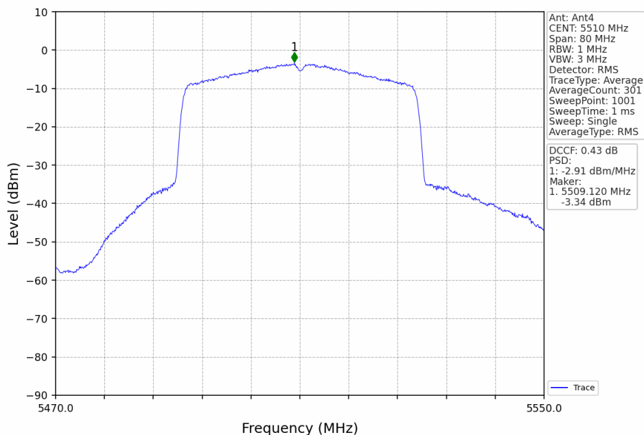
802.11ax(HEW40)_LCH_5510MHz_RU484_Left_Ant4_NTNV
