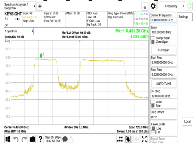
802.11be_80MHz_Chain1_6465MHz_RU484+242_Punc20
