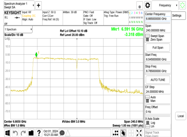
802.11be_160MHz_Chain0_6665MHz_996+484_MRU2
