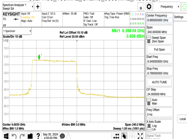
802.11be_160MHz_Chain0_6665MHz_RU996_S67
