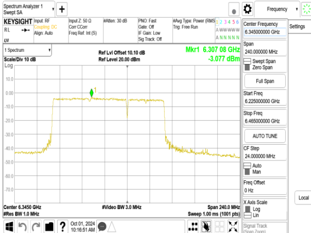
802.11be_160MHz_Chain0_6345MHz_996+484_MRU1
