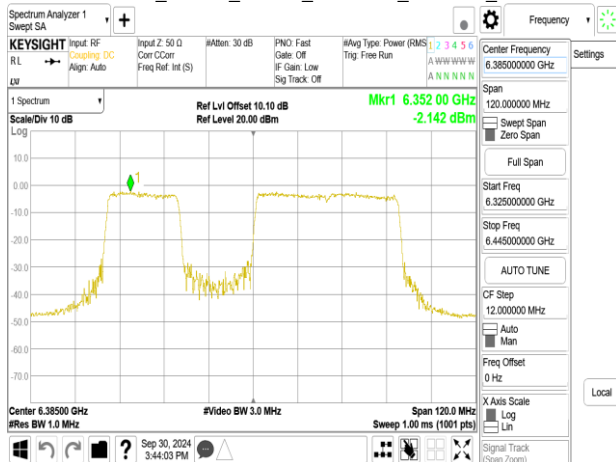
802.11be_80MHz_Chain1_6385MHz_484+242_MRU1
