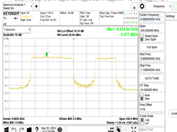
802.11be_160MHz_Chain0_6985MHz_996+484+242_MRU4
