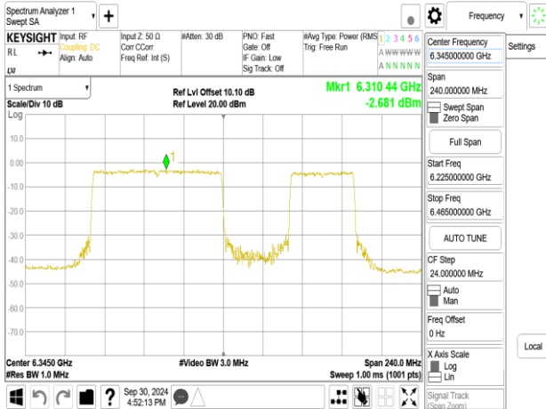
802.11be_160MHz_Chain0_6345MHz_996+484+242_MRU5
