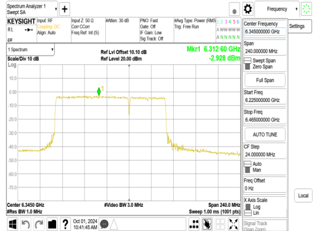
802.11be_160MHz_Chain0_6345MHz_RU996_S67
