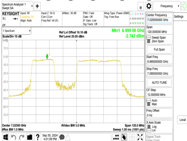
802.11be_80MHz_Chain1_7025MHz_484+242_MR1
