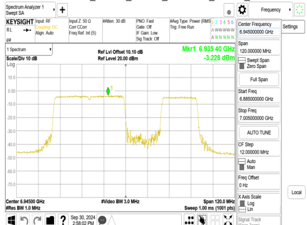
802.11be_80MHz_Chain0_6945MHz_RU484_65
