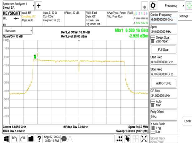
802.11be_160MHz_Chain0_6665MHz_996+484+242_MRU2
