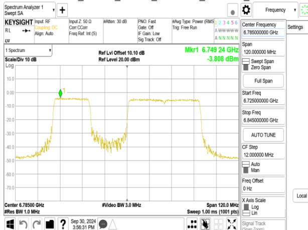
802.11be_80MHz_Chain0_6785MHz_RU484_66
