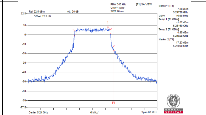
802.11a_Chain 5 / CH48
