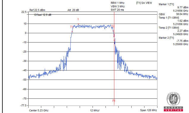
802.11ax (HE40)_Chain 3 / CH46
