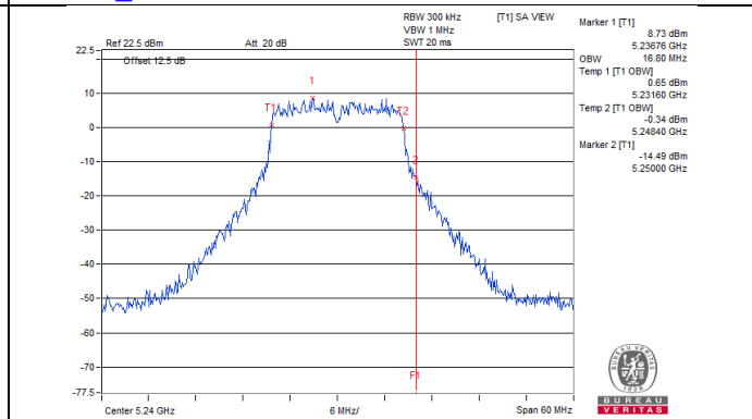
802.11a_Chain 7 / CH48
