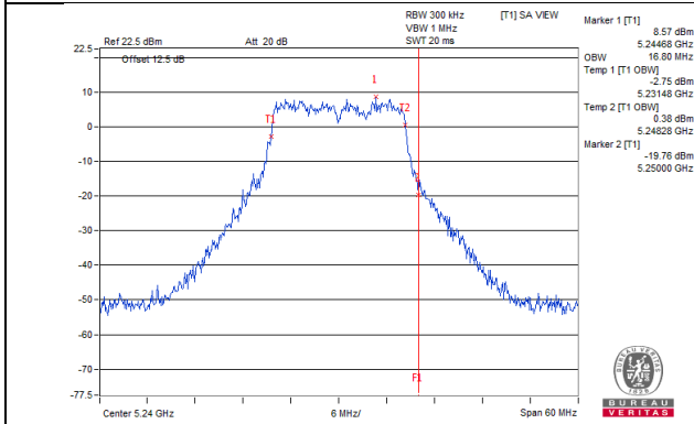
802.11a_Chain 2 / CH48
