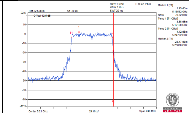
802.11ac (VHT80)_Chain 5 / CH42
