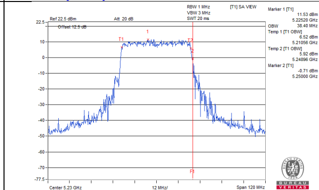
802.11ax (HE40)_Chain 7 / CH46
