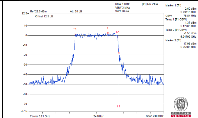
802.11ac (VHT80)_Chain 7 / CH42
