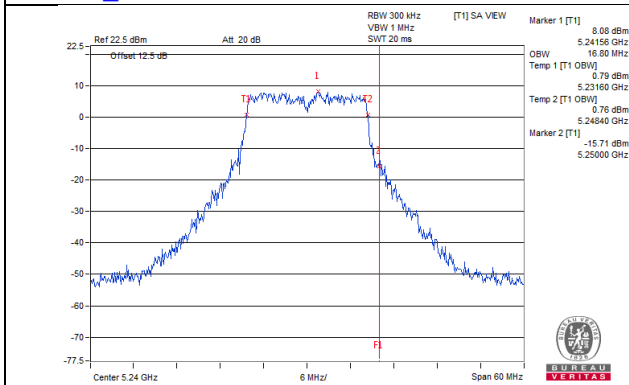
802.11a_Chain 6 / CH48
