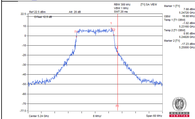
802.11a_Chain 6 / CH48
