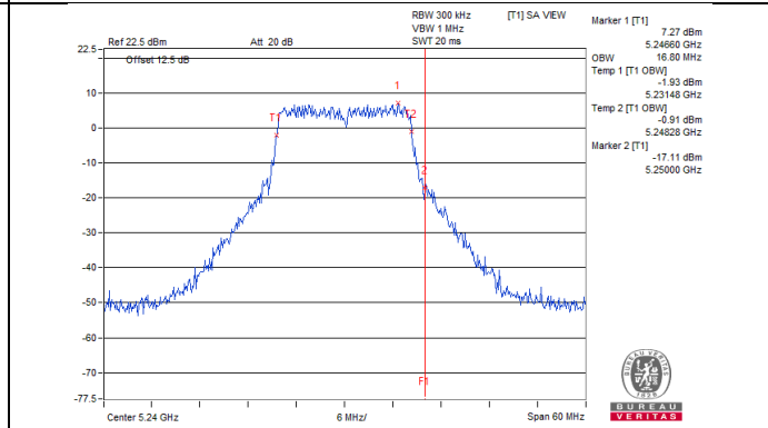
802.11a_Chain 3 / CH48
