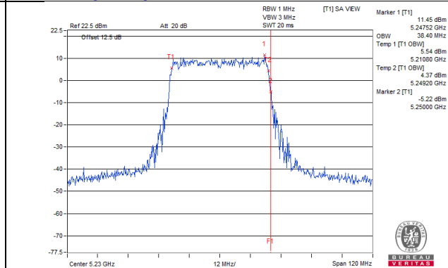
802.11ax (HE40)_Chain 5 / CH46
