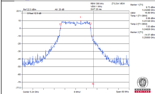
802.11a_Chain 4 / CH48
