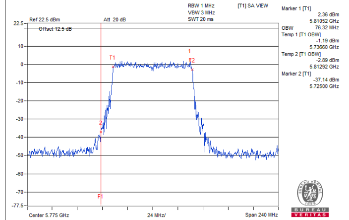
802.11ac (VHT80+80) / Chain 3 : CH155
