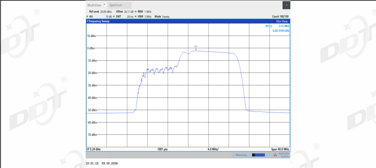
11BE20MIMO_Ant2_5240_52+26_1
