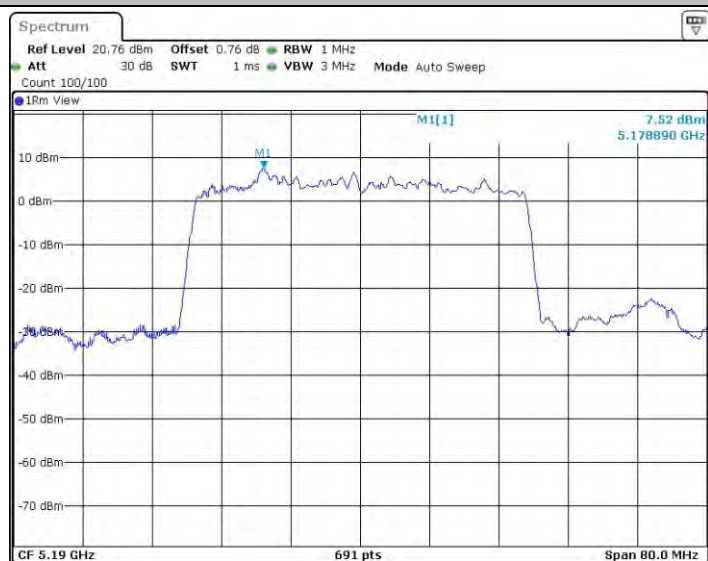
11AX40SISO_Ant0_5190
