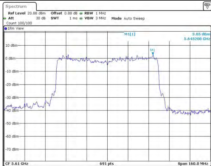
11AX80SISO_Ant0_5610
