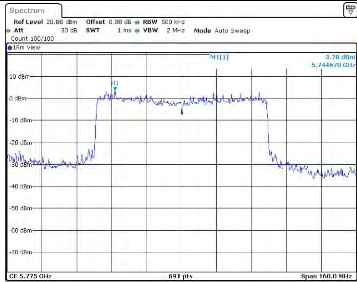
11AX80SISO_Ant0_5775
