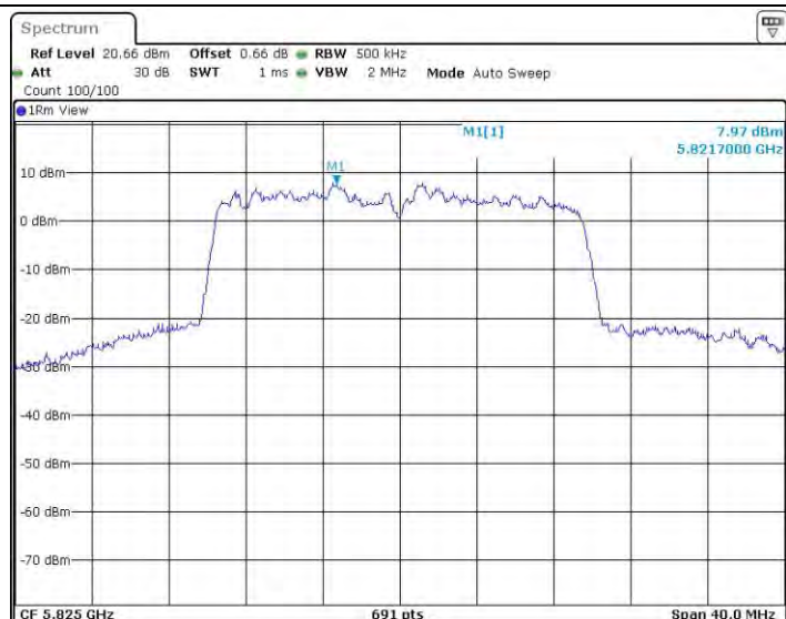
11AX20SISO_Ant0_5825
