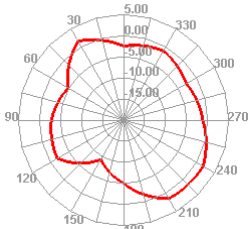
5850.000MHz H
