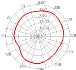
5150.000MHz E2
