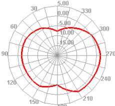
5850.000MHz E2
