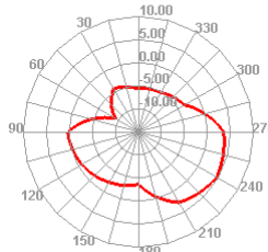
5500.000MHz E1
