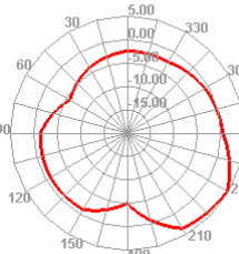
5150.000MHz E1
