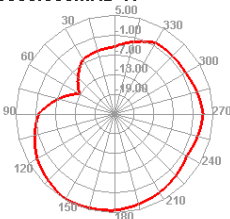
5850.000MHz H
