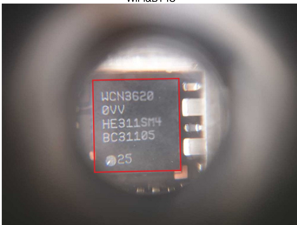
WiFi&BT IC
