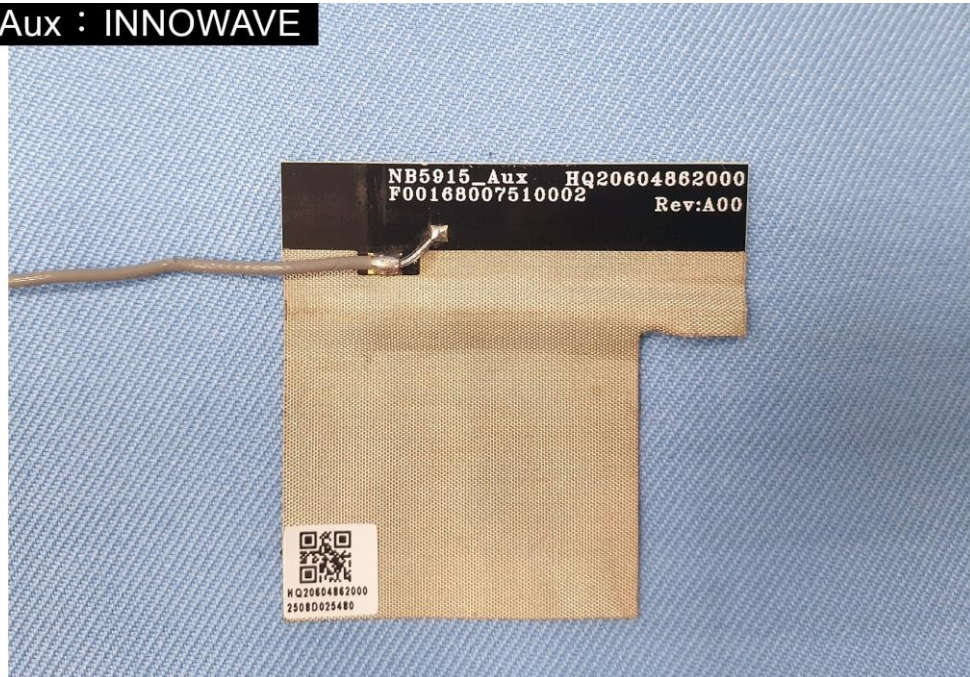
EUT Photo (16)
