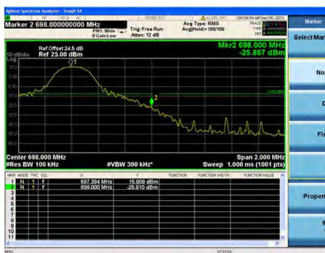
Band71 / 10MHz / High CH / QPSK / 1 RB
