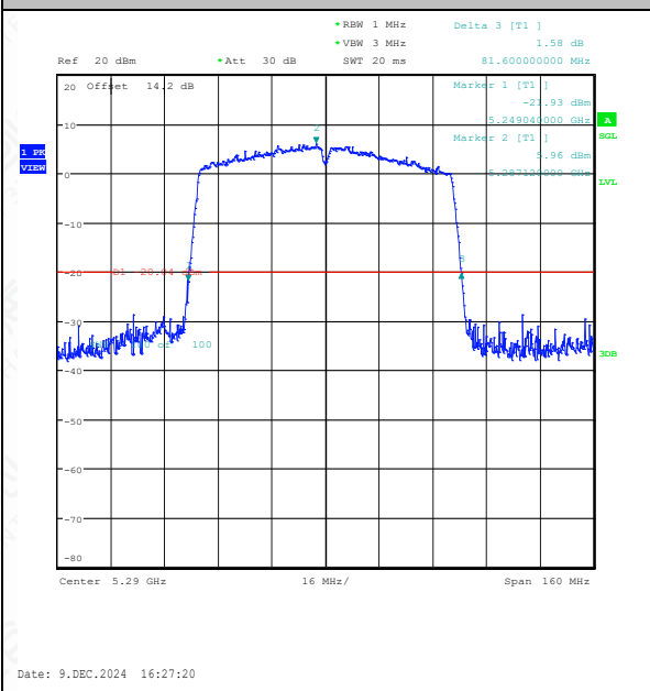
11AC80SISO-Ant1-5290
