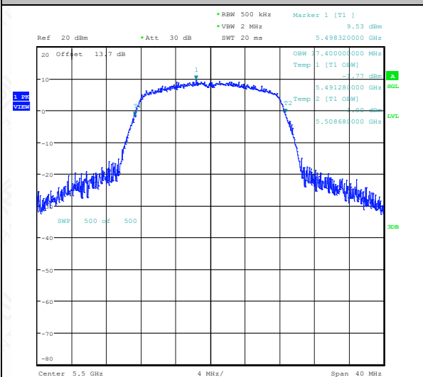
11A-Ant1-5500
