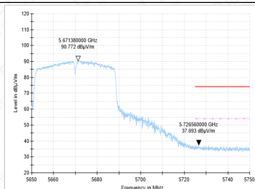
BANDEGE-11AC(40M)-CH134-AV
