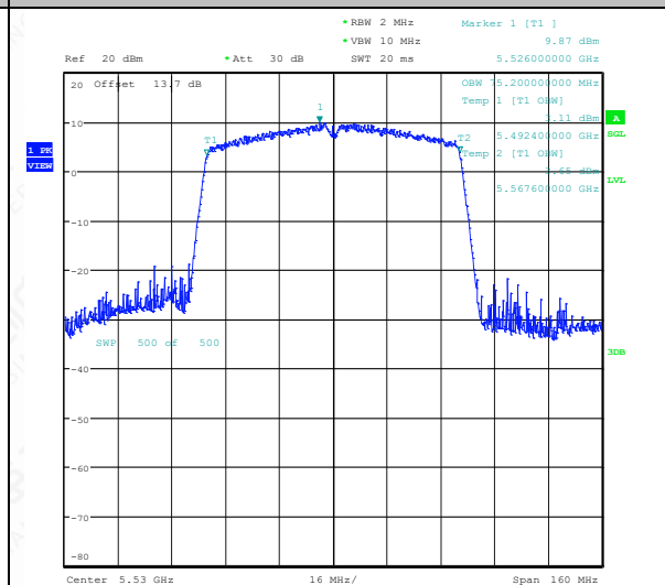
11AC80SISO-Ant1-5530
