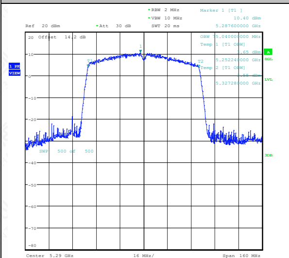
11AC80SISO-Ant1-5290
