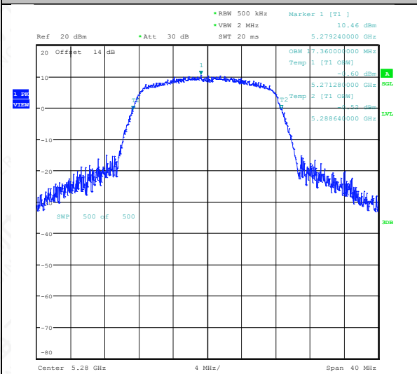
11A-Ant1-5280
