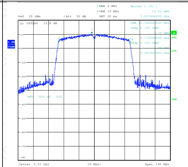
11AC80SISO-Ant1-5210
