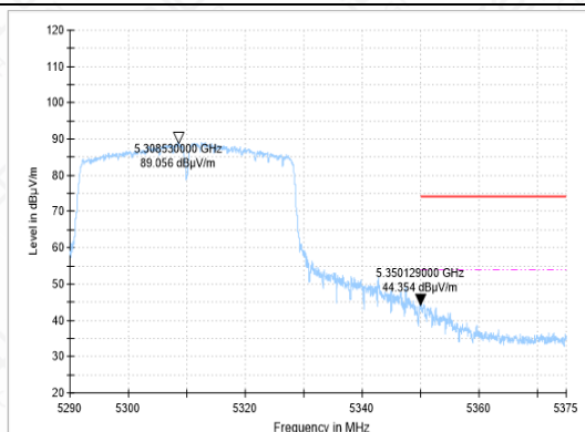
BANDEGE-11AC(40M)-CH62-AV
