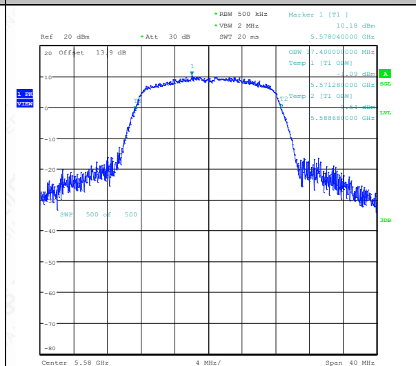
11A-Ant1-5580
