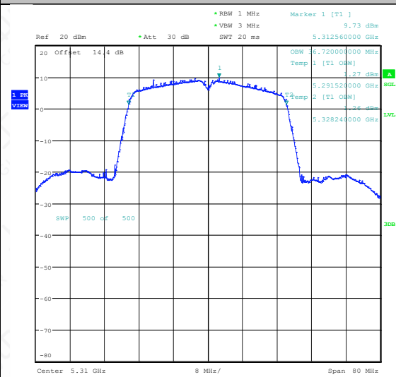
11N40SISO-Ant1-5310
