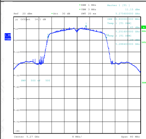
11N40SISO-Ant1-5270
