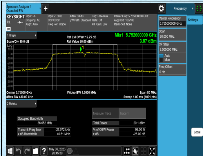
11AC40MIMO-Ant1-5755
