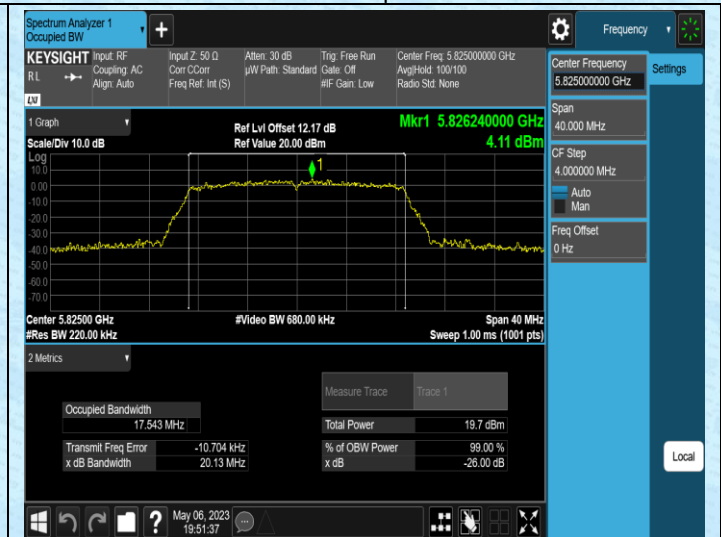
11N20MIMO-Ant1-5825
