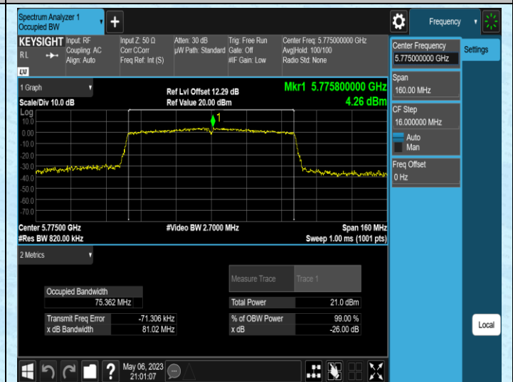
11AC80MIMO-Ant1-5775
