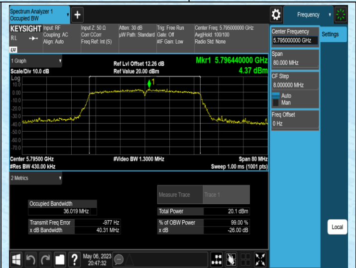
11AC40MIMO-Ant1-5795
