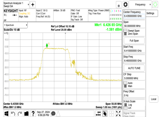
802.11be_20MHz_Chain1_6435MHz_52+26_MRUI
