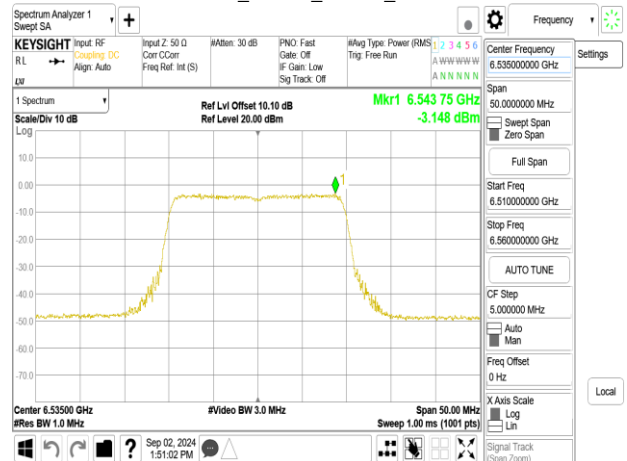
802.11be_20MHz_Chain0_6535MHz_106+26_MRUC1
