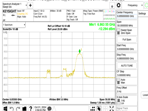
802.11be_20MHz_Chain0_6855MHz_RU52_40
