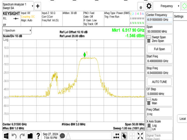
802.11be_20MHz_Chain0_6515MHz_RU106_54
