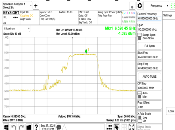
802.11be_20MHz_Chain0_6515MHz_106+26_MRU2
