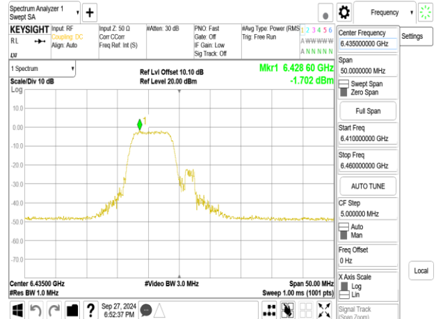
802.11be_20MHz_Chain1_6435MHz_RU106_53
