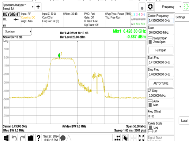
802.11be_20MHz_Chain0_6435MHz_RU26_0
