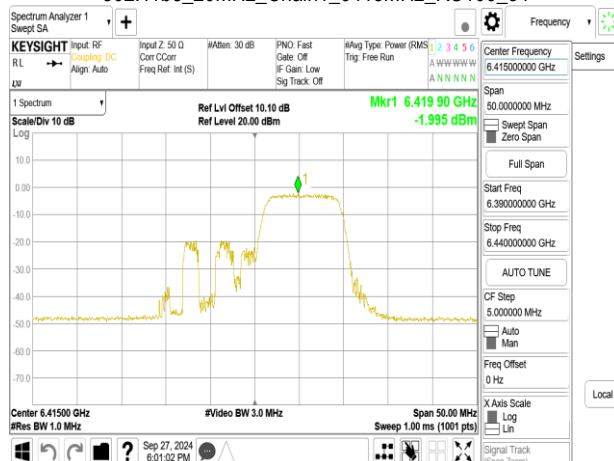
802.11be_20MHz_Chain1_6415MHz_RU106_54
