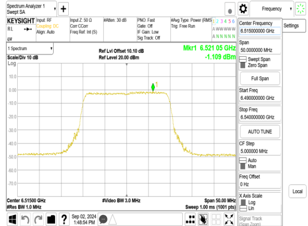
802.11be_20MHz_Chain1_6515MHz_106+26_MRJ2
