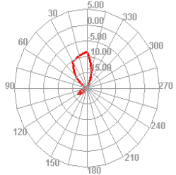
2500.000MHz E2
