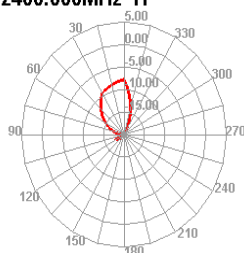
2400.000MHz H
