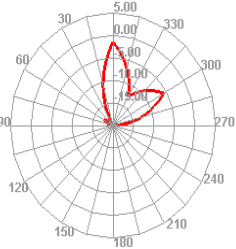
2450.000MHz H
