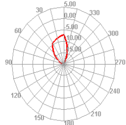
2450.000MHz E2
