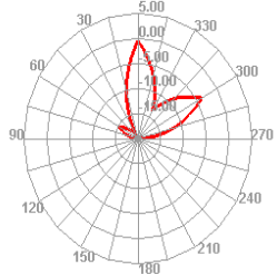
2500.000MHz H
