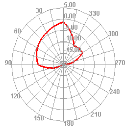
2400.000MHz E1
