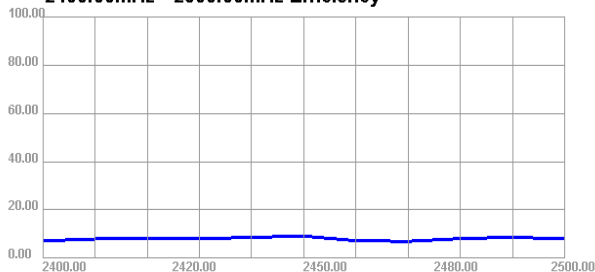
2400.00MHz - 2500.00MHz Efficiency
