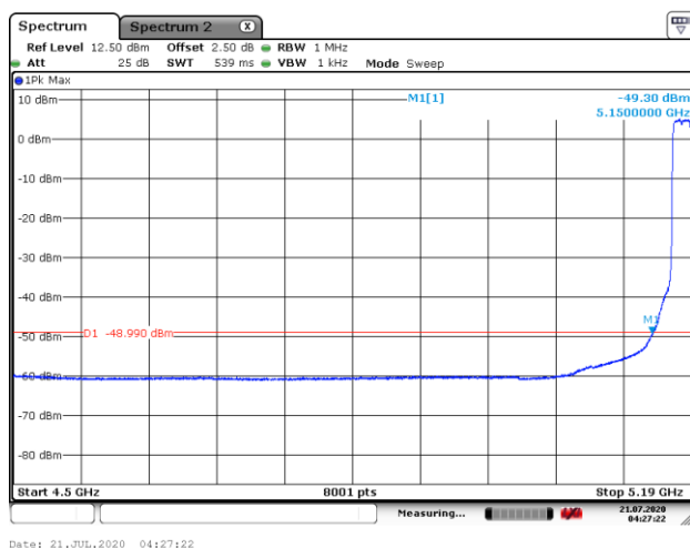
5200MHz with SISO AV
