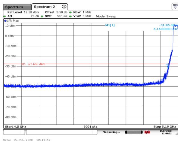
5200MHz PK
