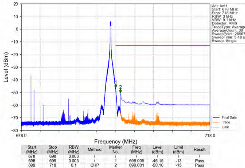
Band71_20MHz_16QAM_HCH_688MHz_RB_1_99_NTNV
