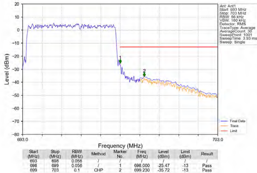
Band71_5MHz_QPSK_HCH_695.5MHz_RB_25_0_NTNV
