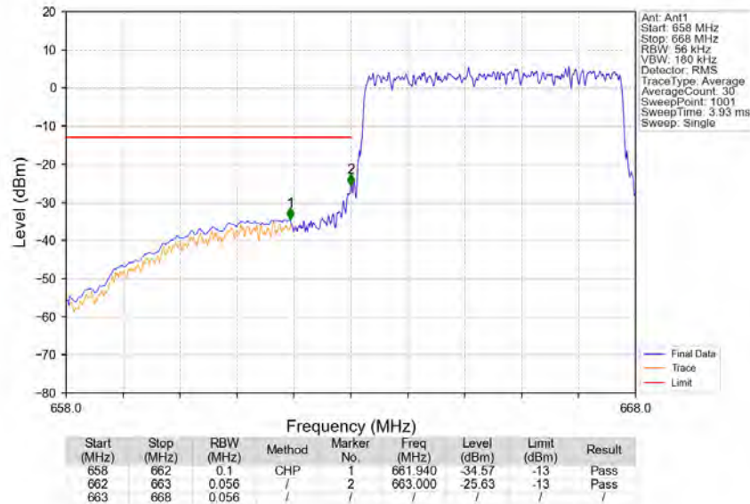
Band71_5MHz_QPSK_LCH_665.5MHz_RB_25_0_NTNV
