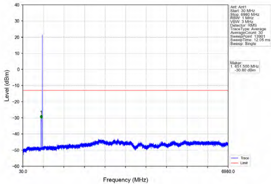
Band71_10MHz_QPSK_HCH_693MHz_RB_1_49_NTNV
