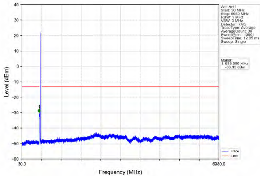
Band71_20MHz_QPSK_HCH_688MHz_RB_1_99_NTNV
