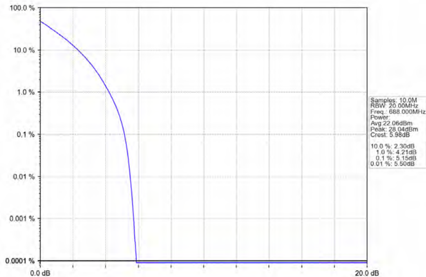
Band71_20MHz_QPSK_HCH_688MHz_RB_100_0_NTNV
