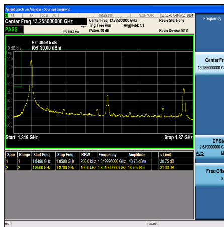
Band2_20MHz_QPSK_18700_1RB#0
