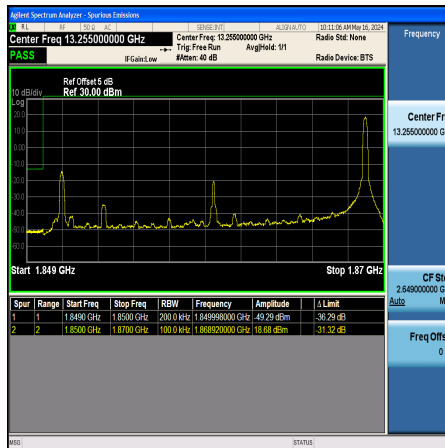
Band2_20MHz_QPSK_18700_1RB#99
