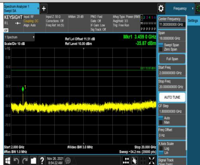
Band4-10MHz-QPSK-20175-50RB#0-Range3:2000~20000MHz
