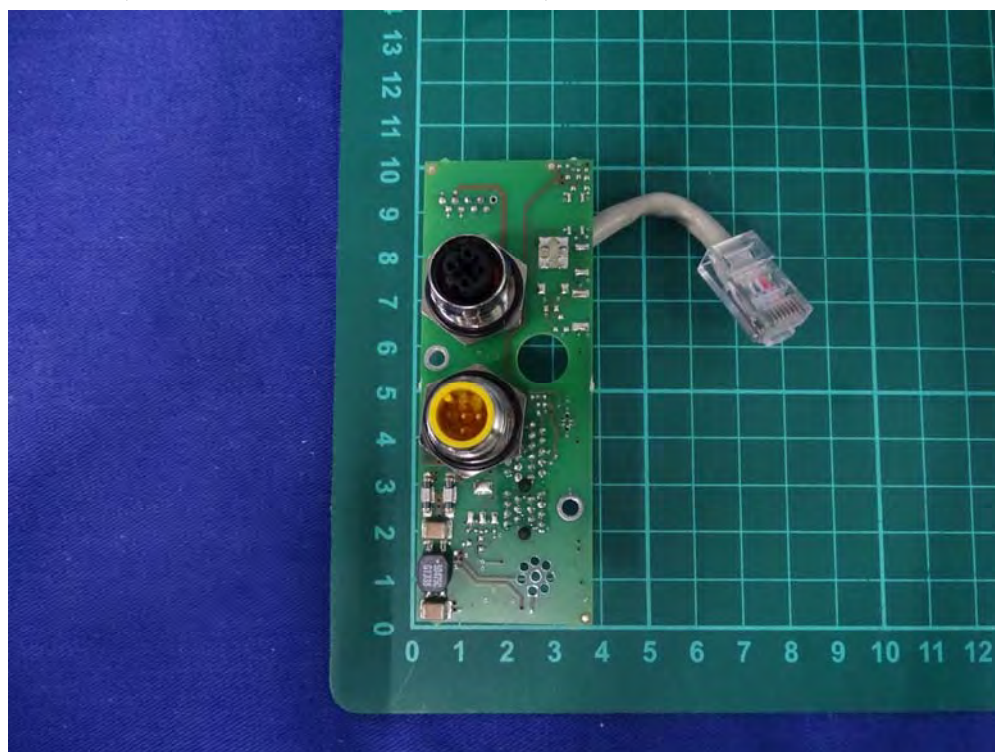
(57) EUT Photo (M/N: BIS U-626-069-111-06-ST31)
