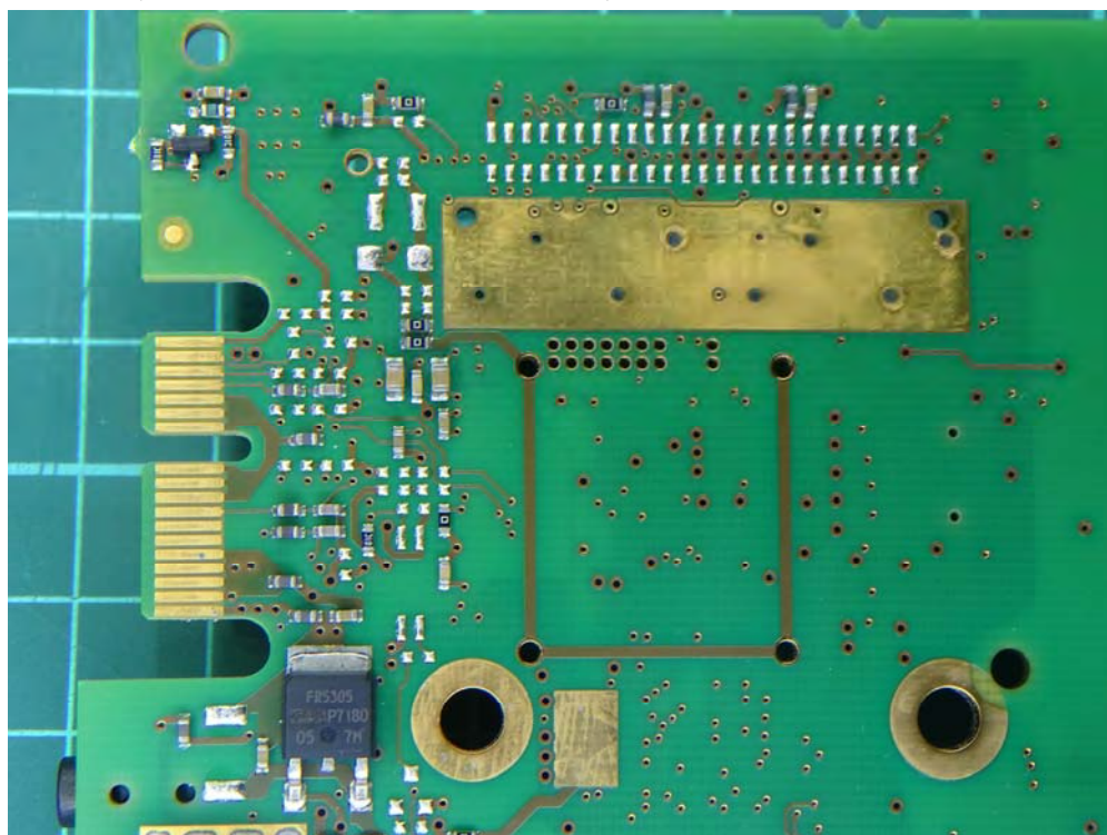
(48) EUT Photo (M/N: BIS U-620-068-111-00-ST29)
