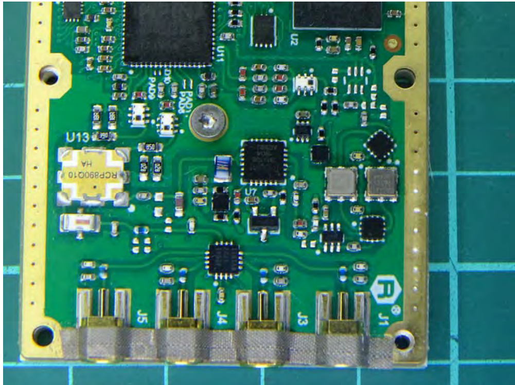
(67) EUT Photo (M/N: BIS U-626-069-111-06-ST31)
