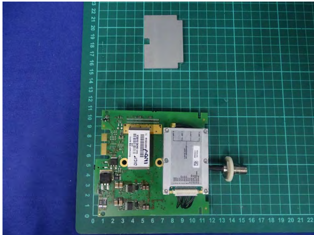
(59) EUT Photo (M/N: BIS U-626-069-111-06-ST31)
