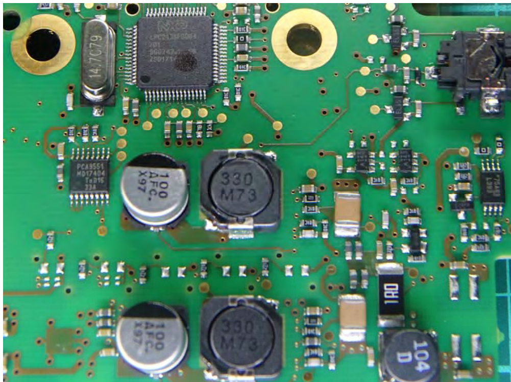
(26) EUT Photo (M/N: BIS U-620-068-111-00-S115)
