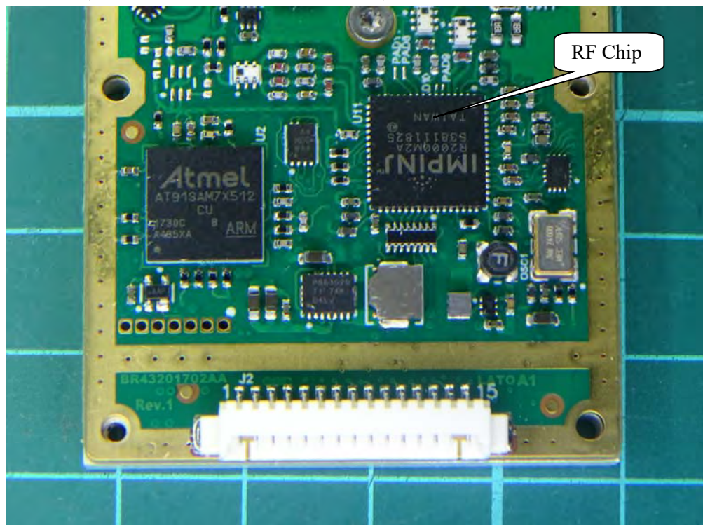
(44) EUT Photo (M/N: BIS U-620-068-111-00-ST29)
