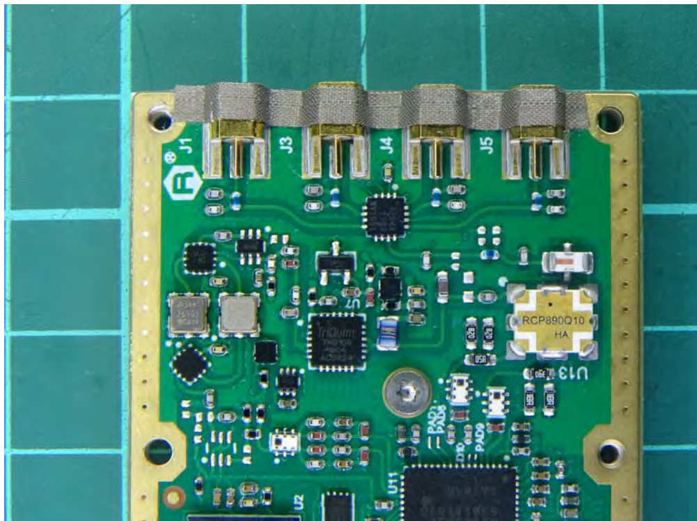
(66) EUT Photo (M/N: BIS U-626-069-111-06-ST31)
