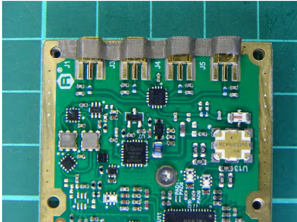
(43) EUT Photo (M/N: BIS U-620-068-111-00-ST29)
