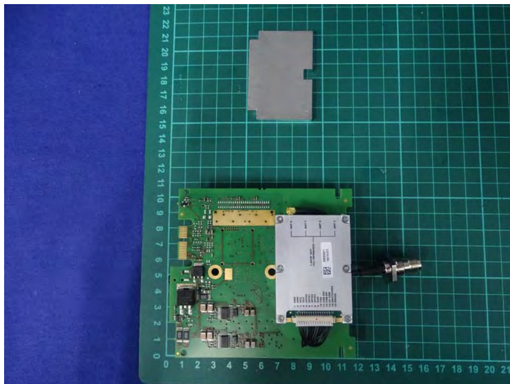
(11) EUT Photo (M/N: BIS U-620-068-111-00-S115)
