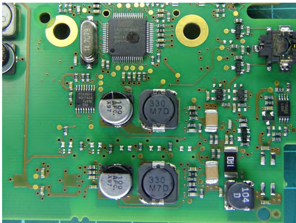
(52) EUT Photo (M/N: BIS U-620-068-111-00-ST29)
