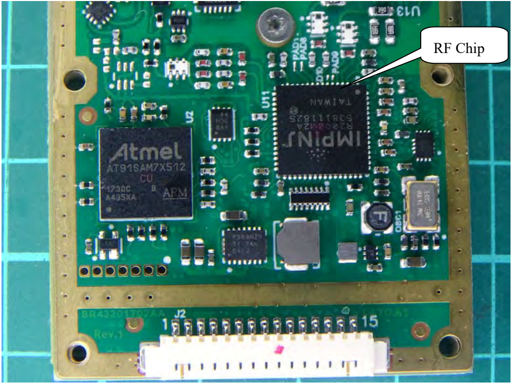
(18) EUT Photo (M/N: BIS U-620-068-111-00-S115)
