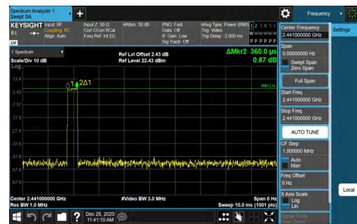
2DH5-Ant0-Hop-PASS
