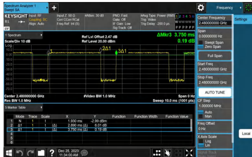
NTNV-3DH5-Ant0-2480
