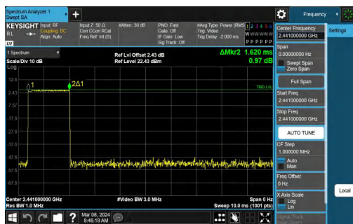
3DH1-Ant0-Hop-PASS
