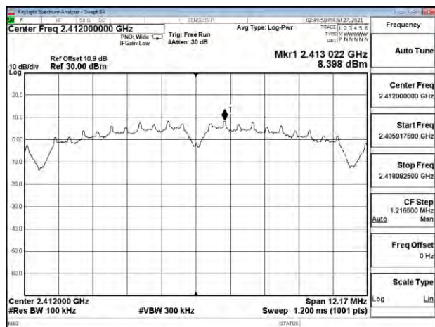
Reference_Level 802.11b_20MHz_Chain0_2412MHz
