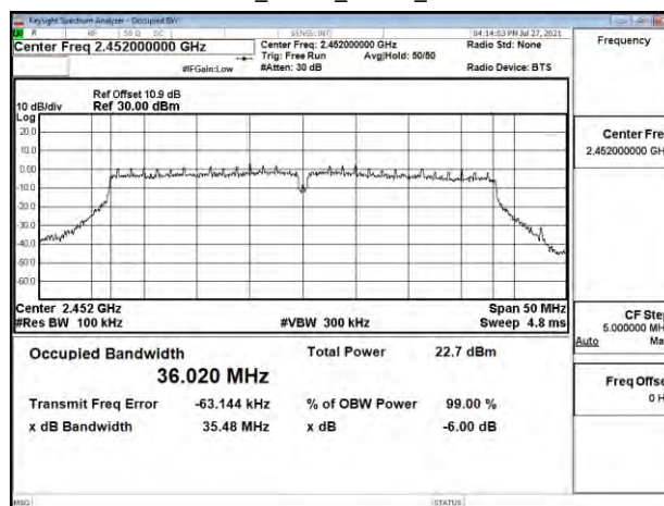
802.11ac_40MHz_Chain1_2452MHz
