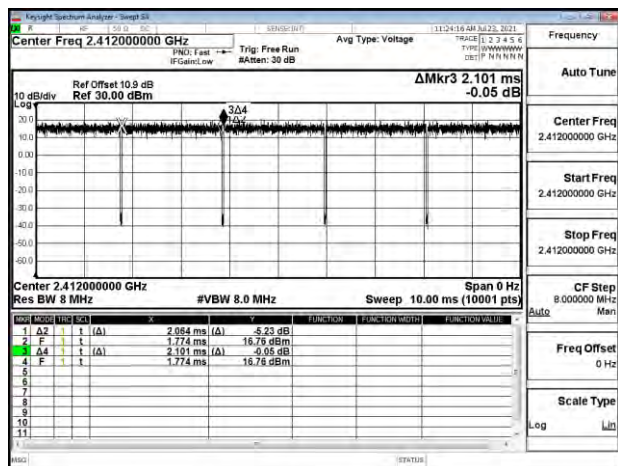
802.11n_20MHz_Chain0_2412MHz
