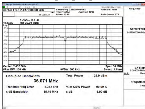
802.11ac_40MHz_Chain0_2437MHz
