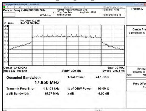
802.11ac_20MHz_Chain1_2462MHz
