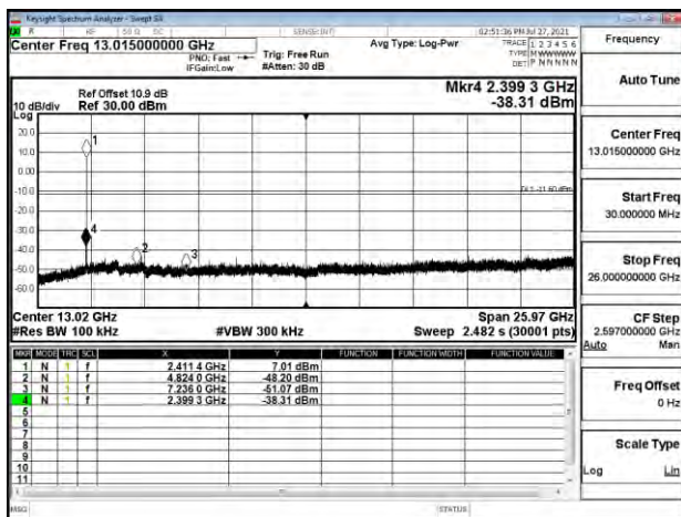
Spurious_Emission 802.11b_20MHz_Chain0_2412MHz
