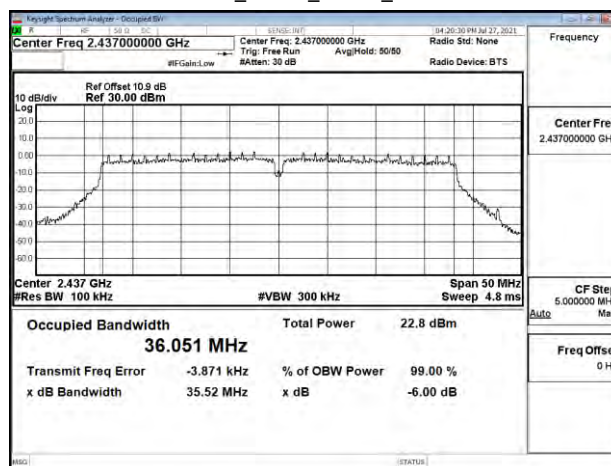
802.11ac_40MHz_Chain1_2437MHz
