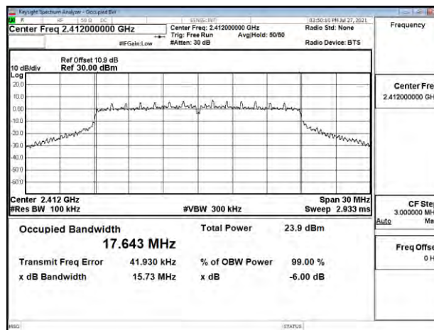
802.11ac_20MHz_Chain1_2412MHz
