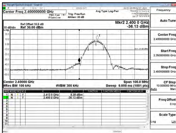
Band_Edge 802.11b_20MHz_Chain0_2412MHz
