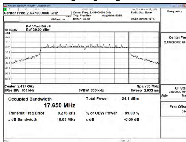
802.11ac_20MHz_Chain1_2437MHz
