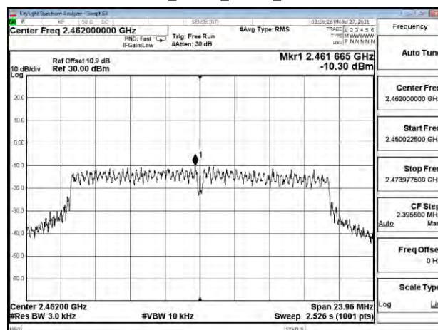
802.11ac_20MHz_Chain1_2462MHz
