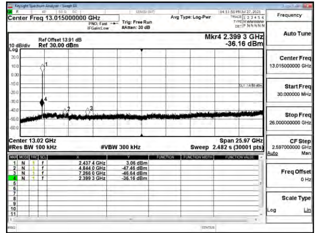
802.11ac_40MHz_Chain0_2437MHz
