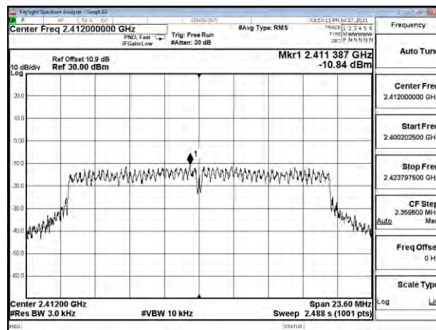
802.11ac_20MHz_Chain1_2412MHz
