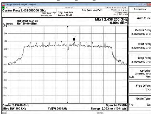
802.11ac_20MHz_Chain0_2437MHz
