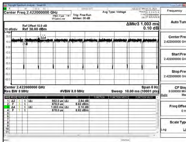
802.11ac_40MHz_Chain0_2422MHz
