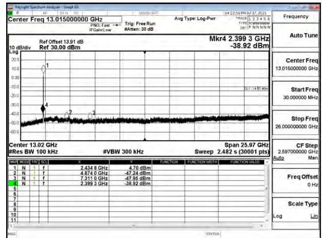
802.11ac_40MHz_Chain0_2437MHz
