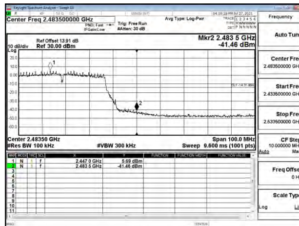
802.11ac_40MHz_Chain0_2452MHz
