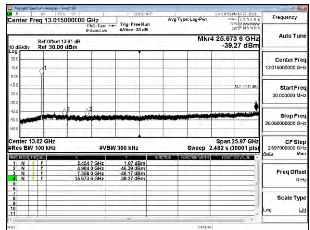
802.11ac_40MHz_Chain0_2452MHz
