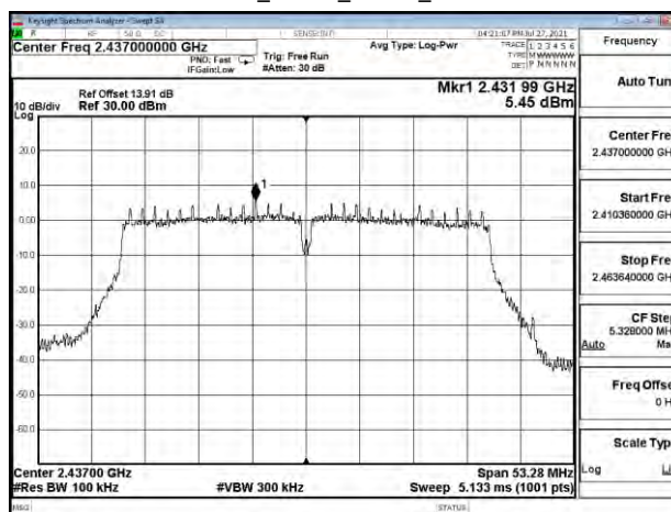
802.11ac_40MHz_Chain0_2437MHz
