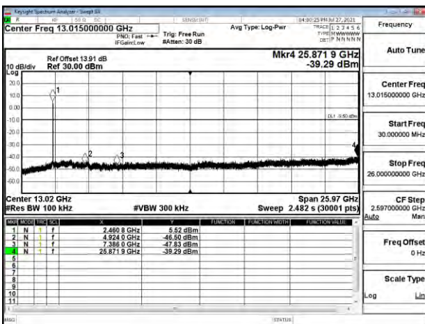
802.11ac_20MHz_Chain0_2462MHz
