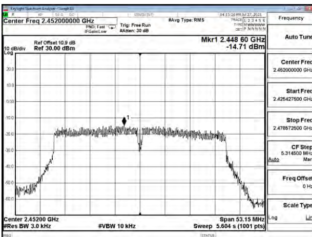
802.11ac_40MHz_Chain0_2452MHz
