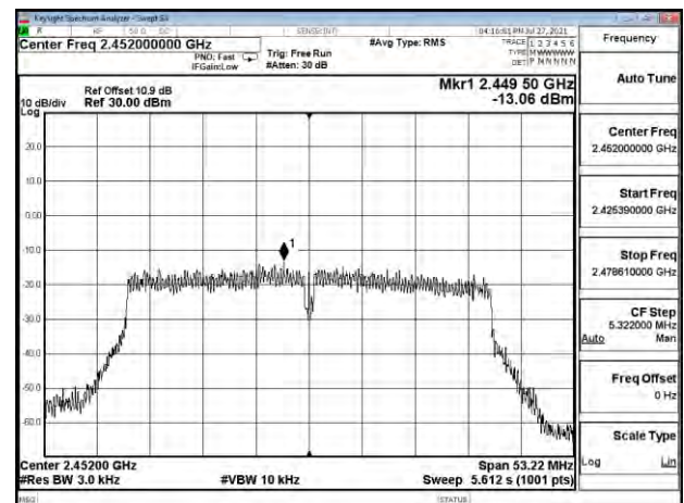
802.11ac_40MHz_Chain1_2452MHz
