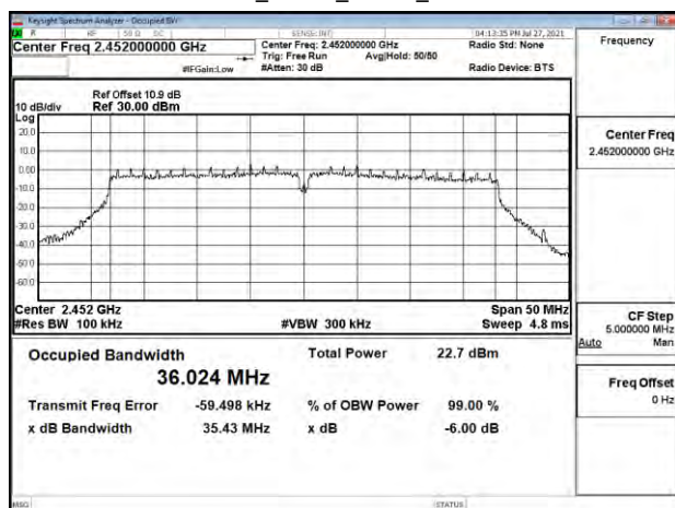
802.11ac_40MHz_Chain0_2452MHz
