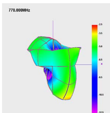
E1 plane
