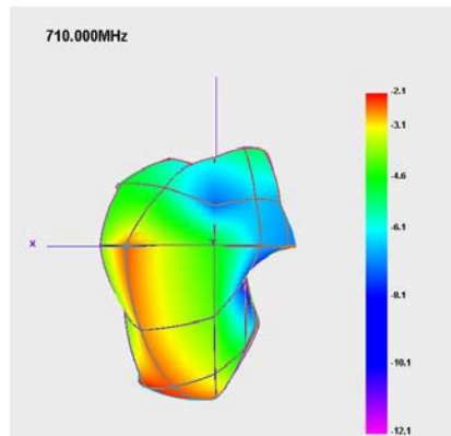
E2 plane
