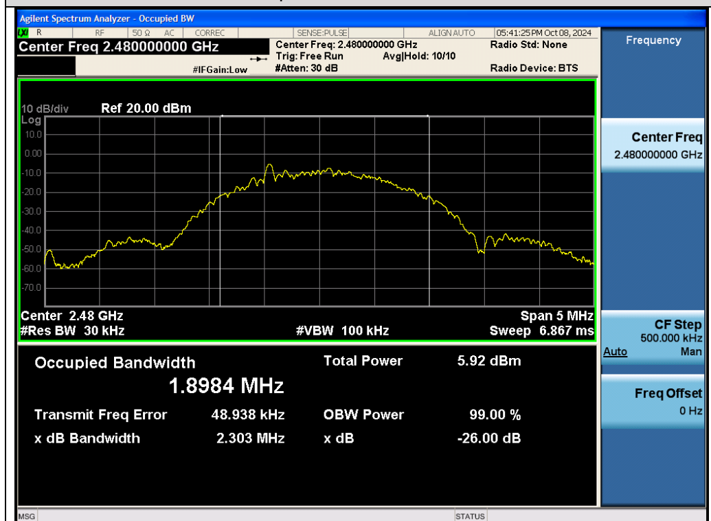
Test_Graph_2.4G_ANT1_2480_OBW
