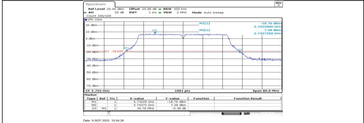
11AC40MIMO_Ant2_5755
