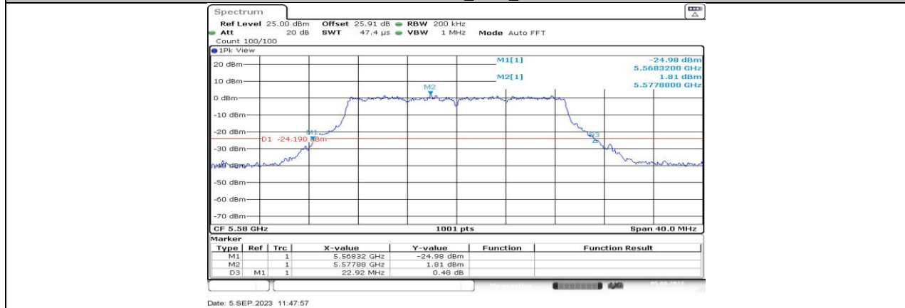
11AC20MIMO_Ant2_5580
