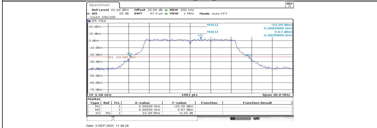
11AC20MIMO_Ant3_5580
