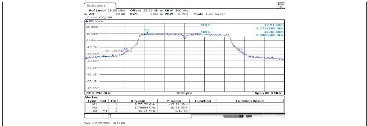
11AC40MIMO_Ant4_5795
