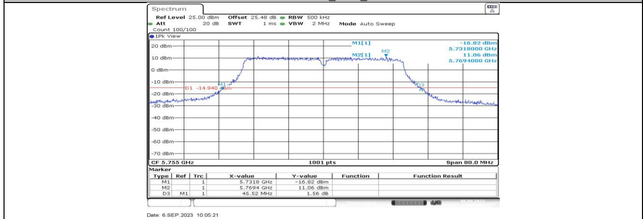
11AC40MIMO_Ant3_5755
