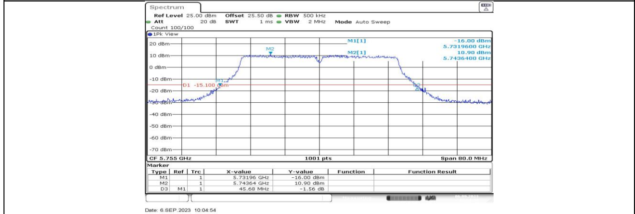
11AC40MIMO_Ant3_5755
