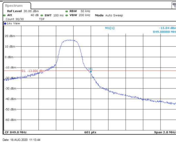
Band5-3MHz-QPSK-20635-1RB#0
