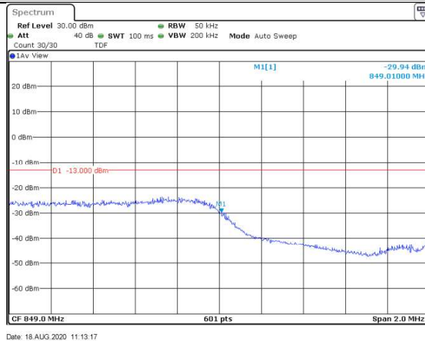
Band5-3MHz-QPSK-20635-15RB#0
