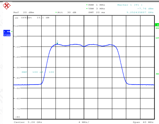
11AX20MIMO-Ant1-5260-PASS
