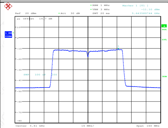
11AC80SISO-Ant2-5610-PASS
