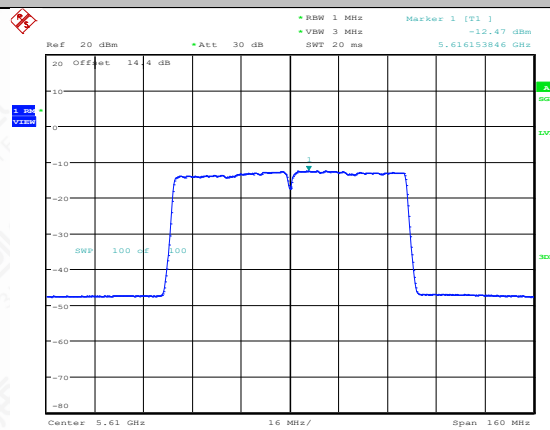
11AC80SISO-Ant1-5610-PASS
