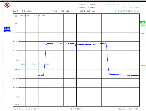
11AC80SISO-Ant2-5530-PASS
