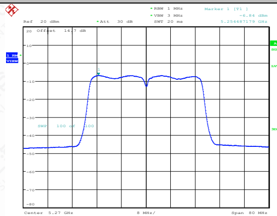
11N40SISO-Ant1-5270-PASS
