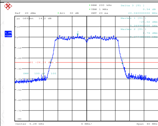
11N20MIMO-Ant2-5280
