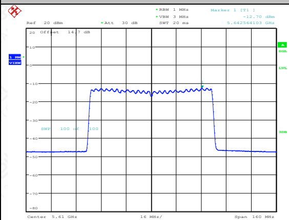
11AX80SISO-Ant2-5610-PASS
