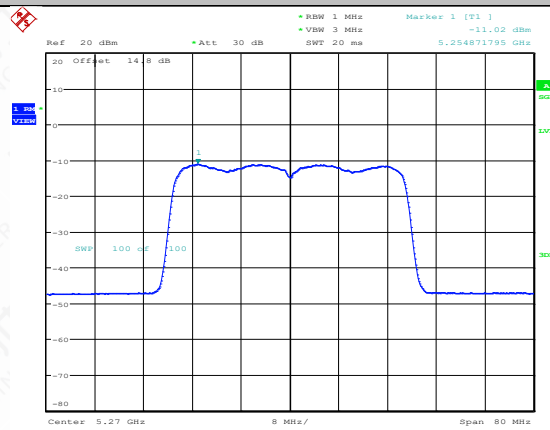
11AX40MIMO-Ant1-5270-PASS
