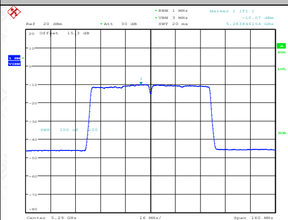
11AC80SISO-Ant2-5290-PASS
