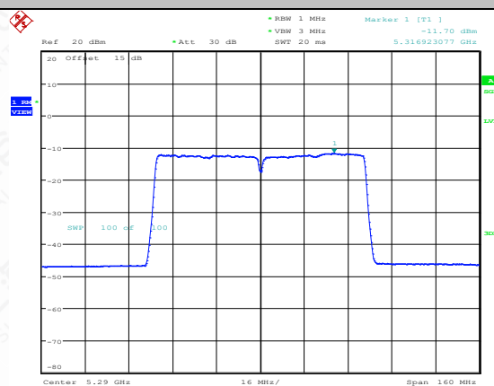
11AC80SISO-Ant1-5290-PASS
