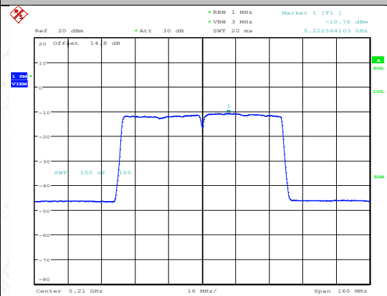
11AC80SISO-Ant2-5210-PASS
