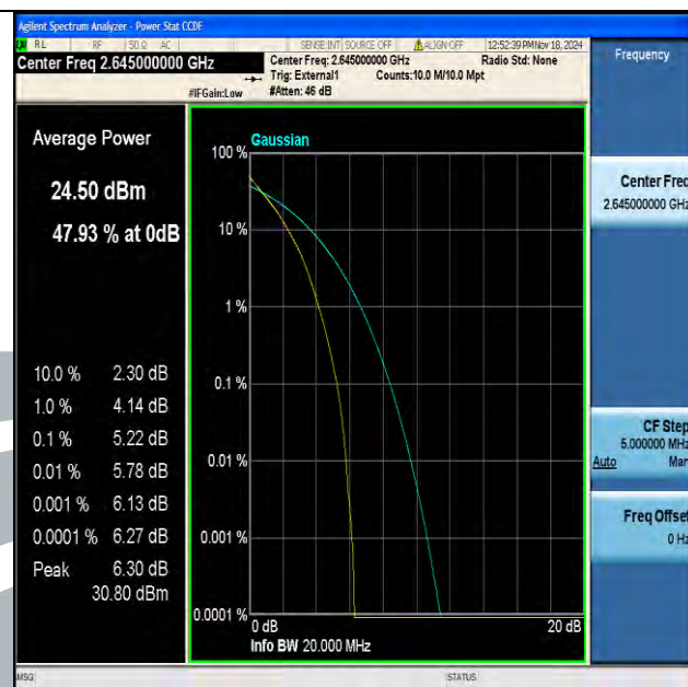
Band41(2535-2655)-20MHz-QPSK-41140-100RB#0-PASS
