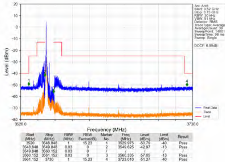
n78d_30kHz_SISO_NTNV_10MHz_DFT-s-OFDM PI/2 BPSK_3555MHz_Inner_1RB_Left
