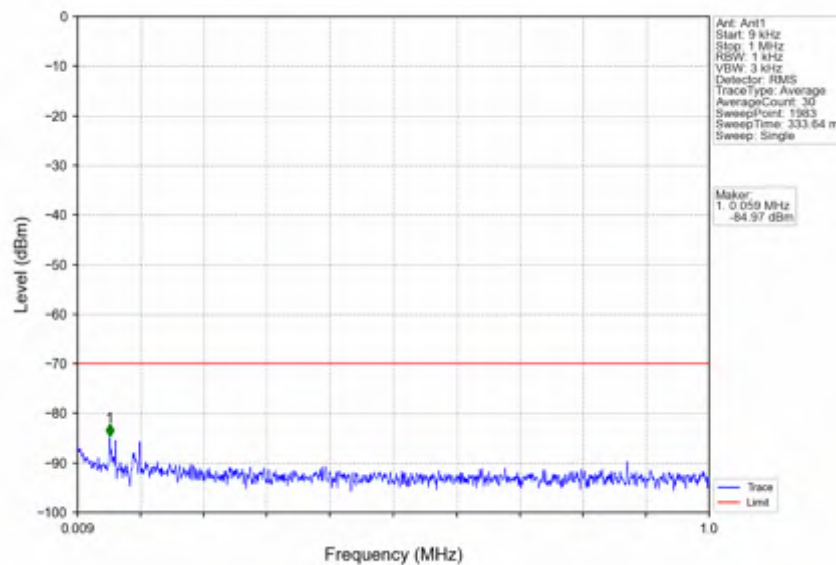
n78d_30kHz_SISO_NTNV_10MHz_DFT-s-OFDM PI/2 BPSK_3555MHz_Inner_1RB_Left
