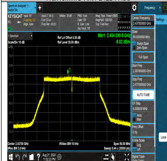
11ax40MIMO-Ant1-2437-PASS
