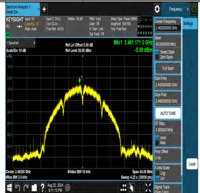
11b-CDD-Ant2-2462-PASS
