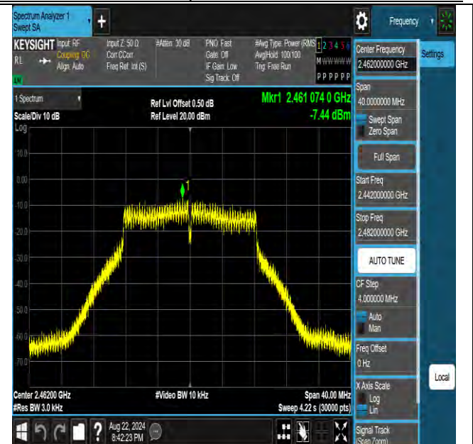
11g-CDD-Ant2-2462-PASS
