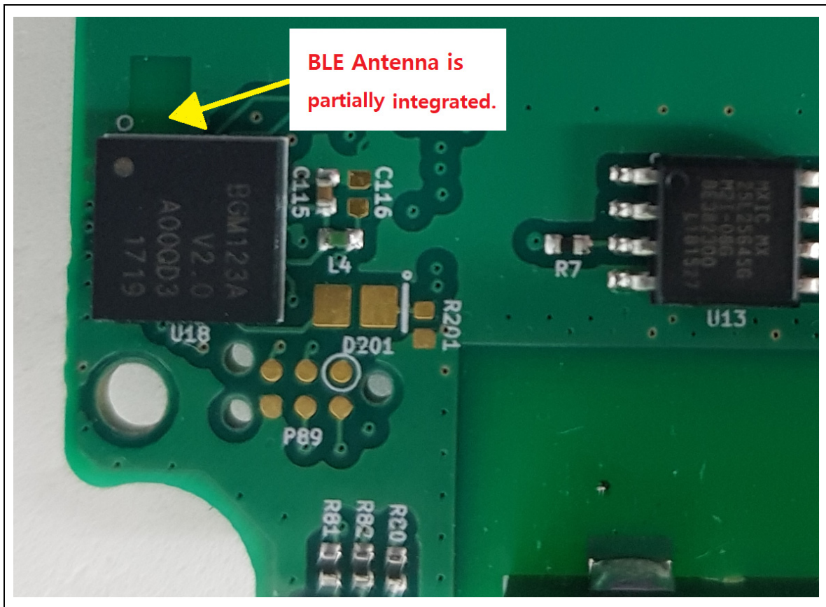
&lt;Bluetooth LE Antenna&gt;
