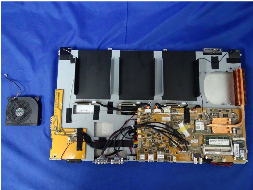
(82) EUT Photo
