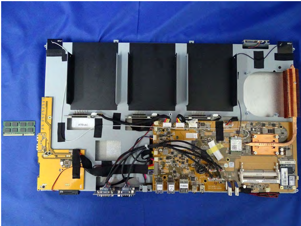
(91) EUT Photo
