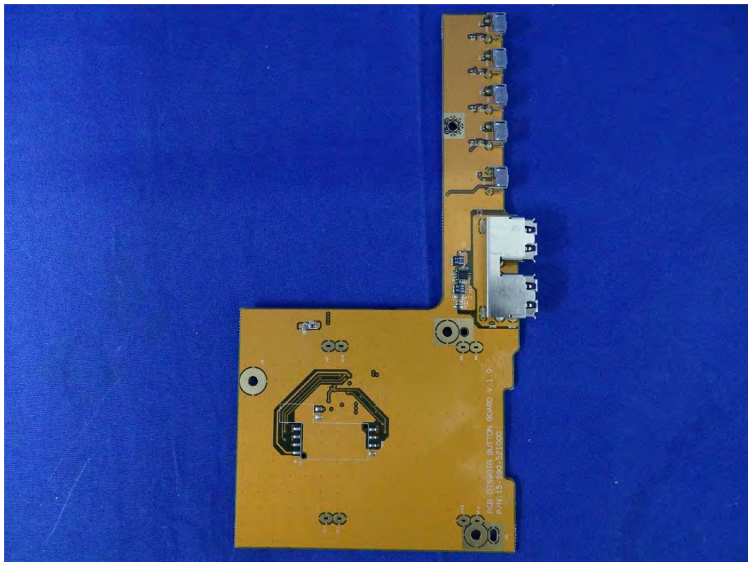
(88) EUT Photo
