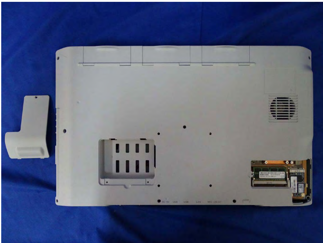
(78) EUT Photo
