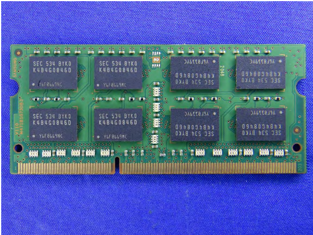
(93) EUT Photo
