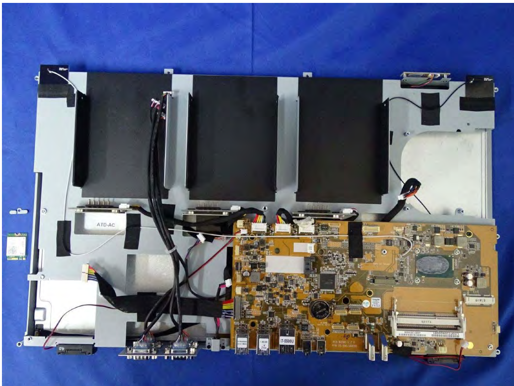
(98) EUT Photo
