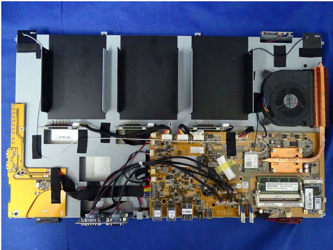
(81) EUT Photo
