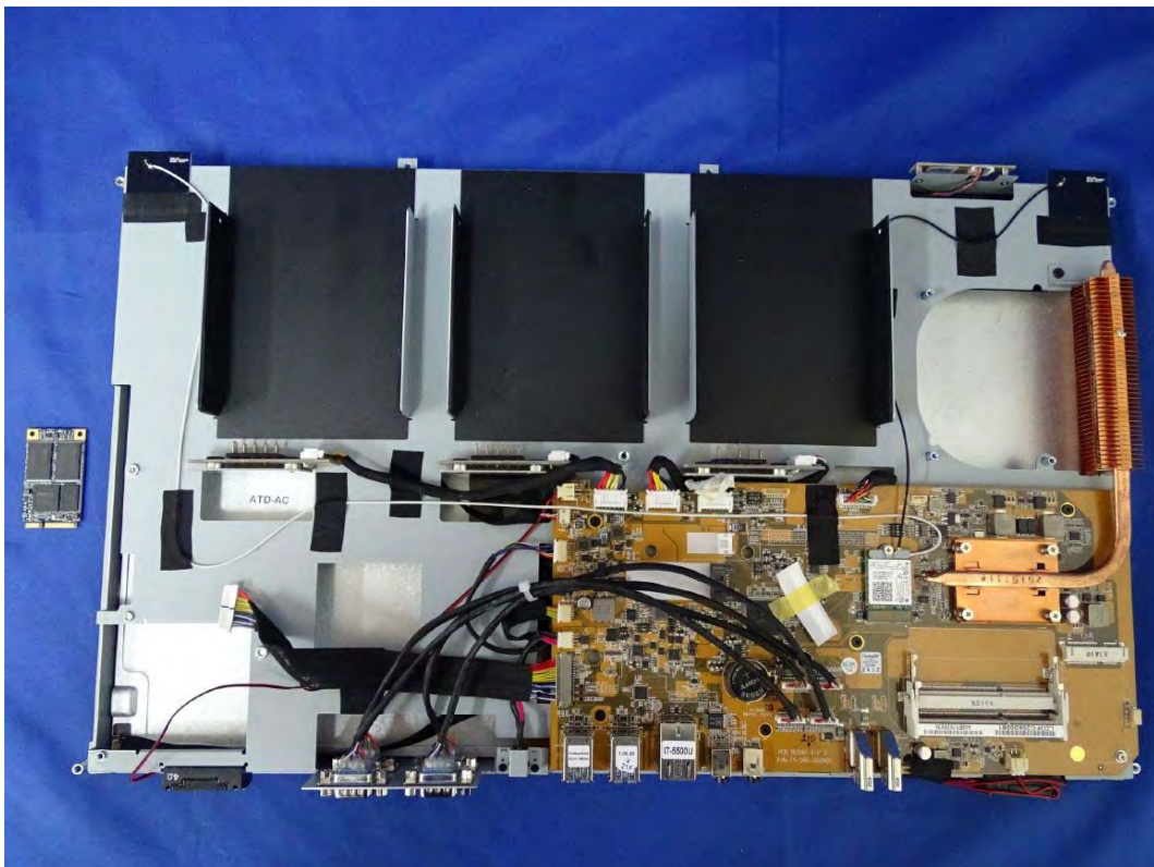
(94) EUT Photo
