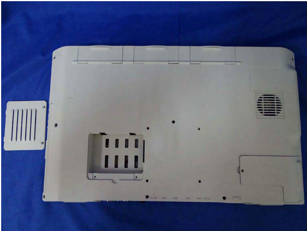
(77) EUT Photo
