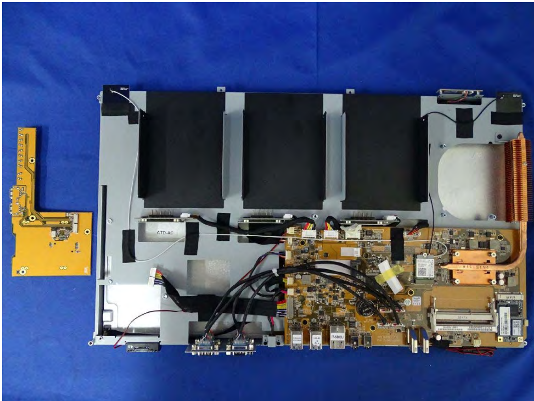
(85) EUT Photo
