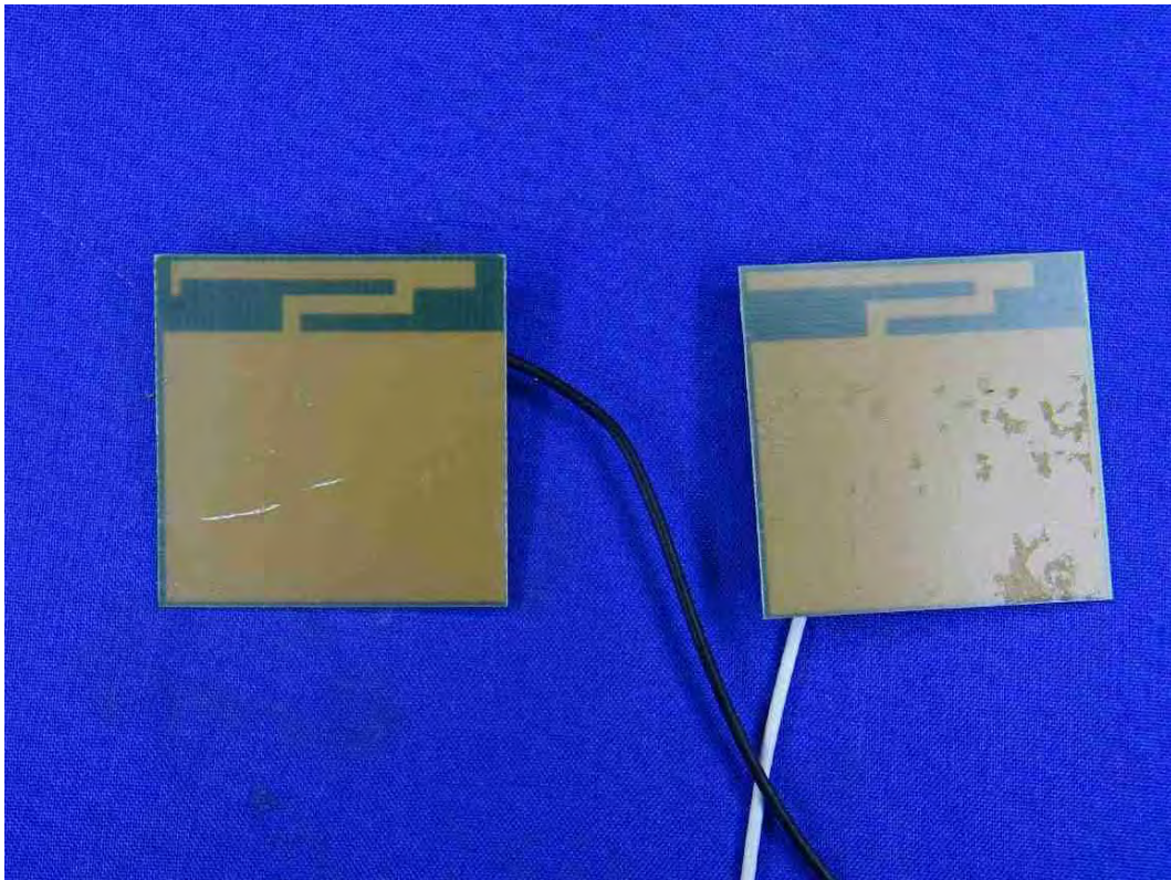
(62) EUT Photo
