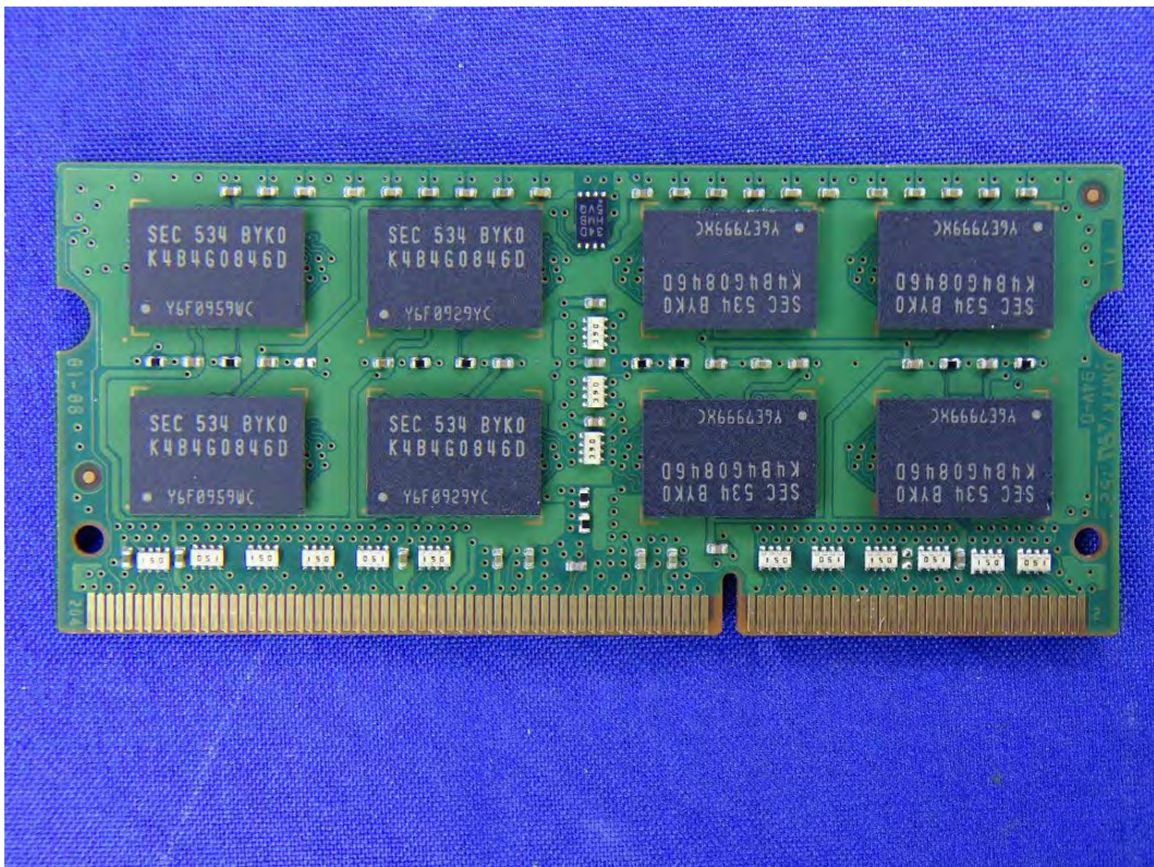
(92) EUT Photo
