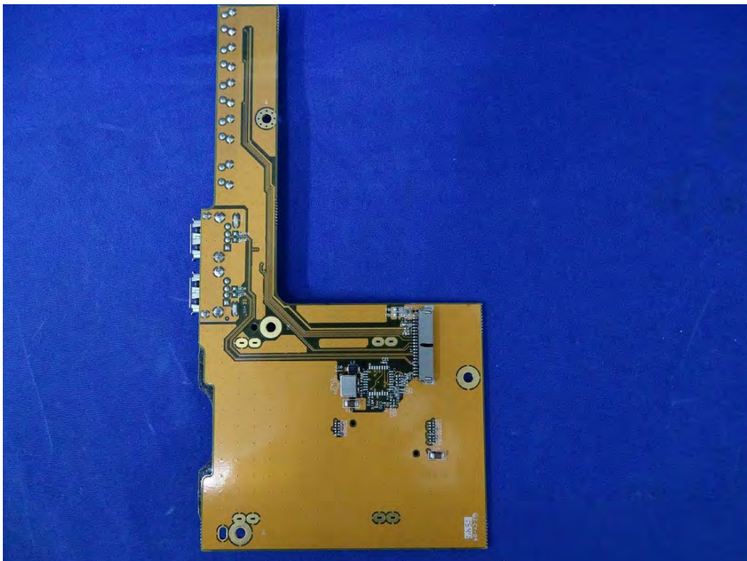
(86) EUT Photo
