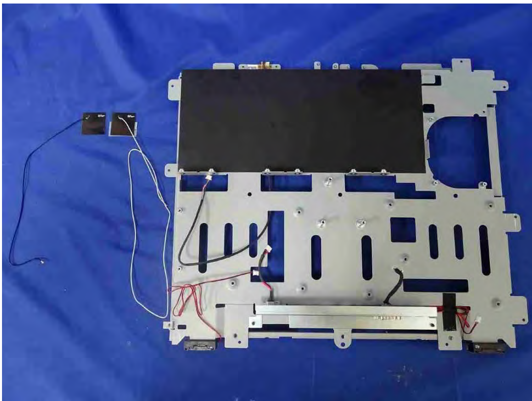
(59) EUT Photo
