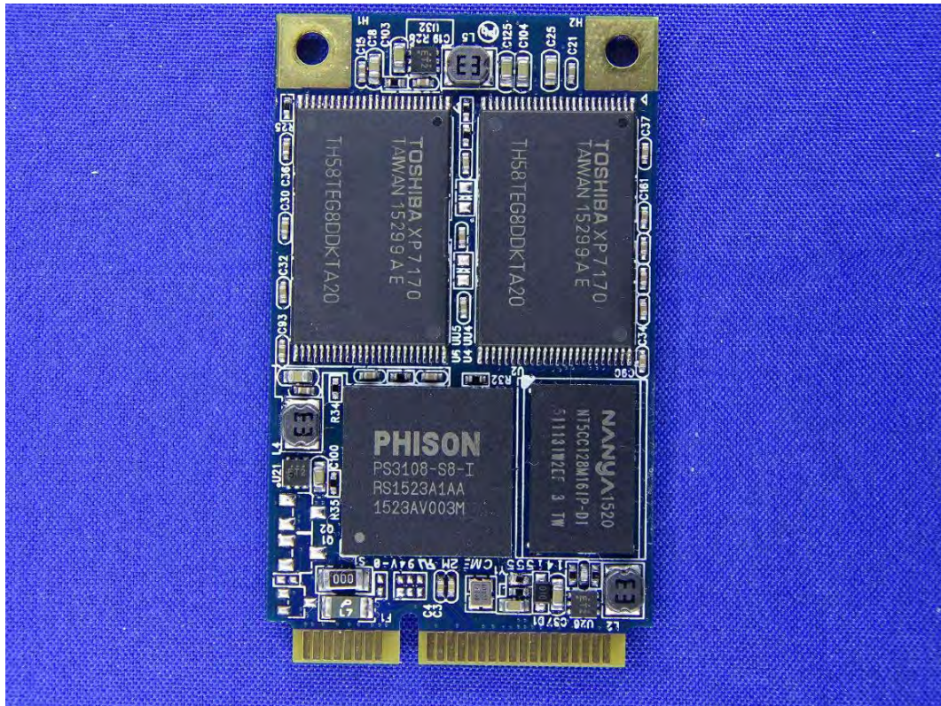
(95) EUT Photo
