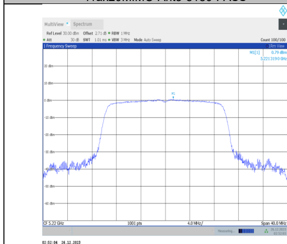
11ax20MIMO-Ant1-5220-PASS
