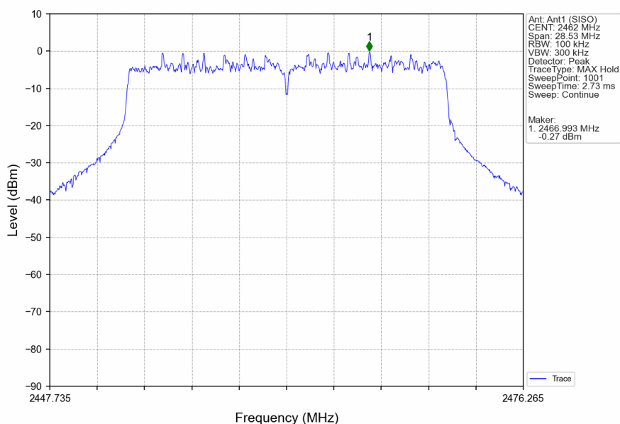
802.11ax(HEW20)_HCH_2462MHz_SU_/_Ant1 (SISO)_NTNV
