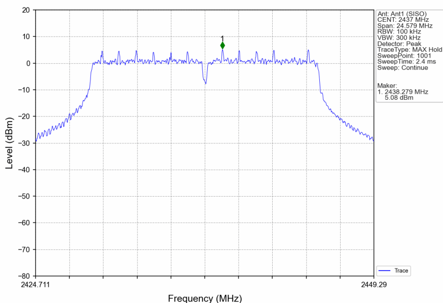
802.11g_MCH_2437MHz_Ant1 (SISO)_NTNV
