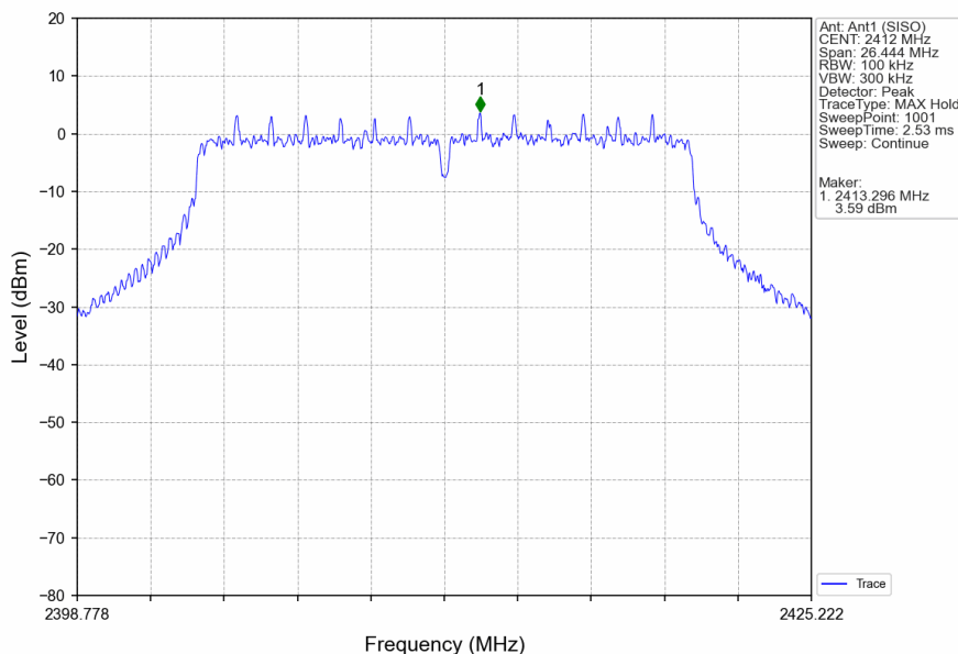
802.11n(HT20)_LCH_2412MHz_Ant1 (SISO)_NTNV
